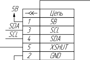
A14 VL53LOX
