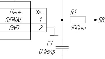
A1 концевик
