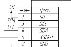
A15 VL53LOX
