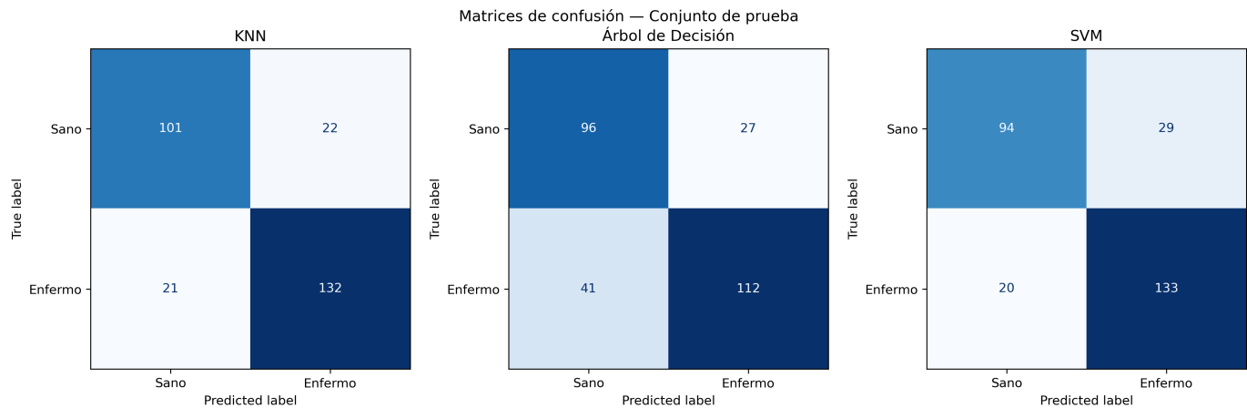
Figura 18: Matrices de confusión sobre el conjunto de prueba de Heart Disease.
