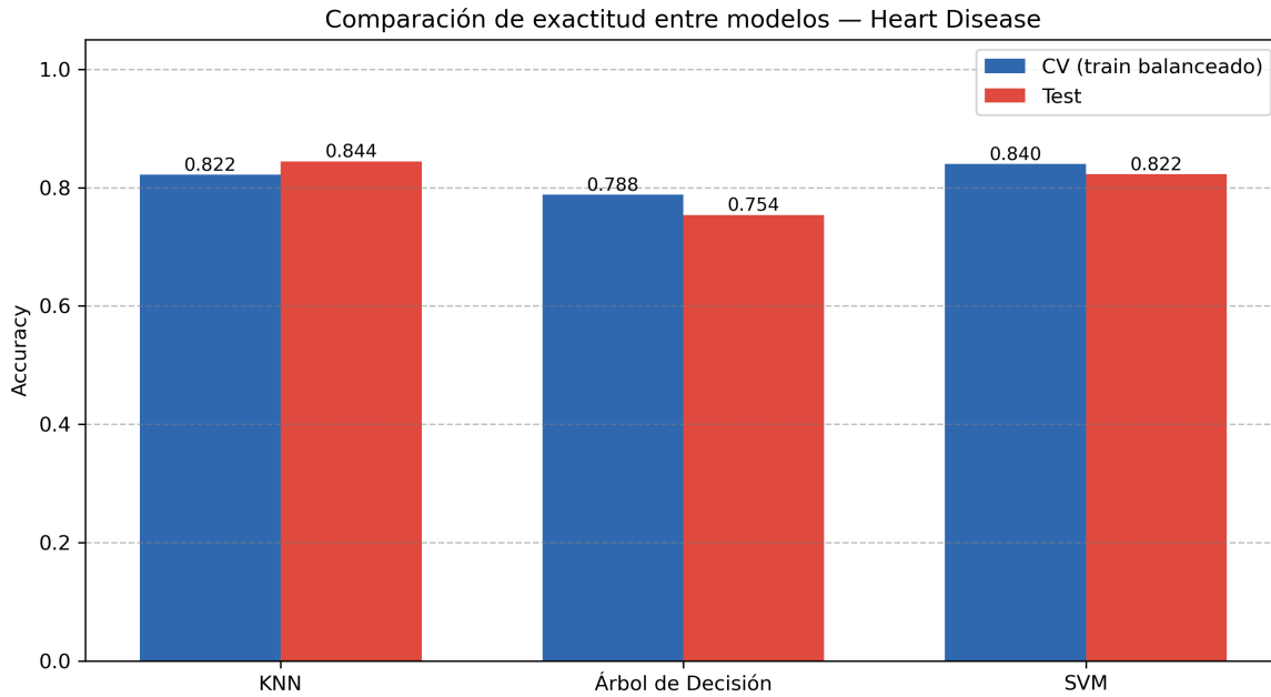
Figura 21: Comparación de exactitud CV vs Test sobre Heart Disease.
