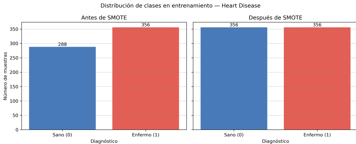
Figura 14: Distribución de clases en train de Heart Disease antes y después de SMOTE.
