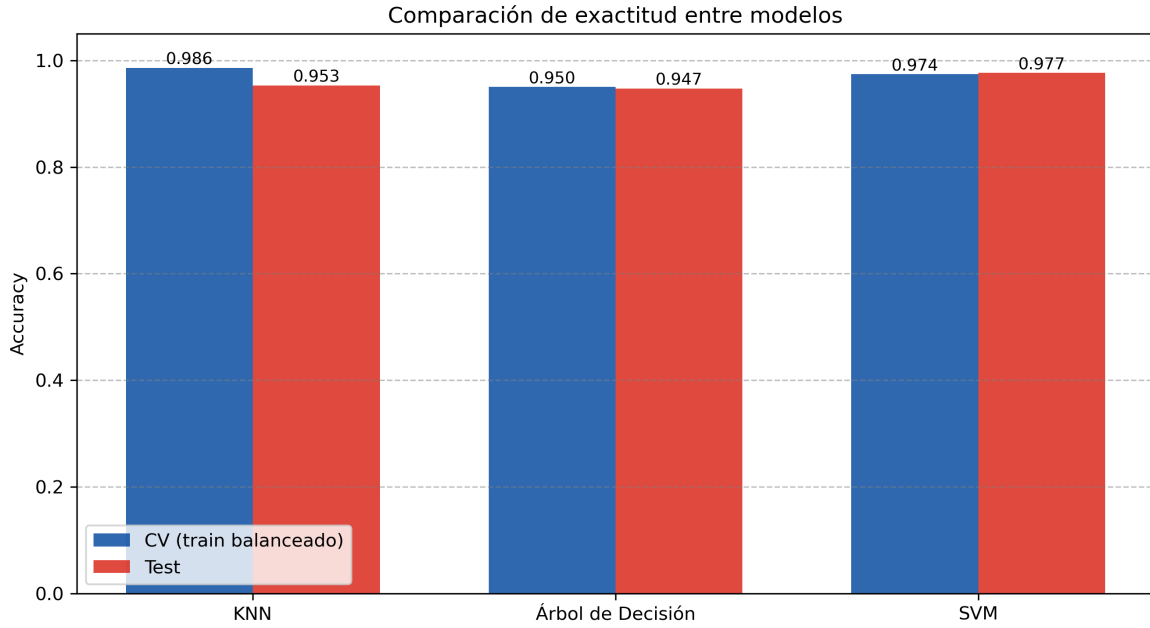
Figura 11: Comparación de exactitud CV vs Test para los tres modelos sobre Cancer.
