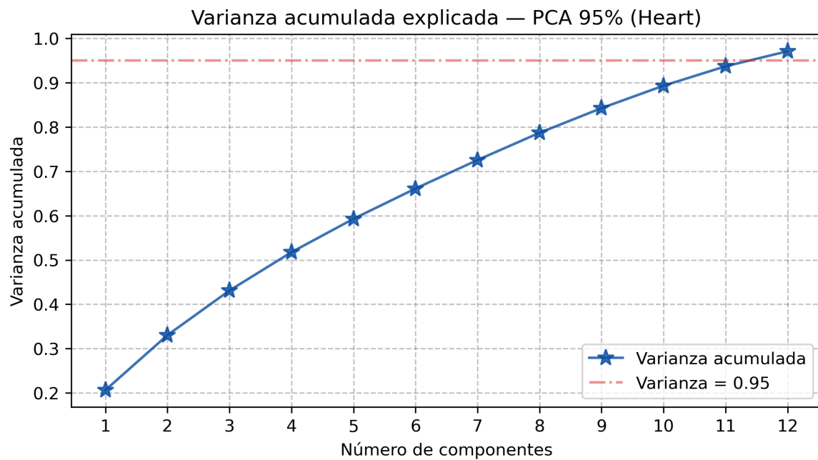
Figura 16: Varianza acumulada al fijar PCA con 95 %: se requieren 12 componentes.
