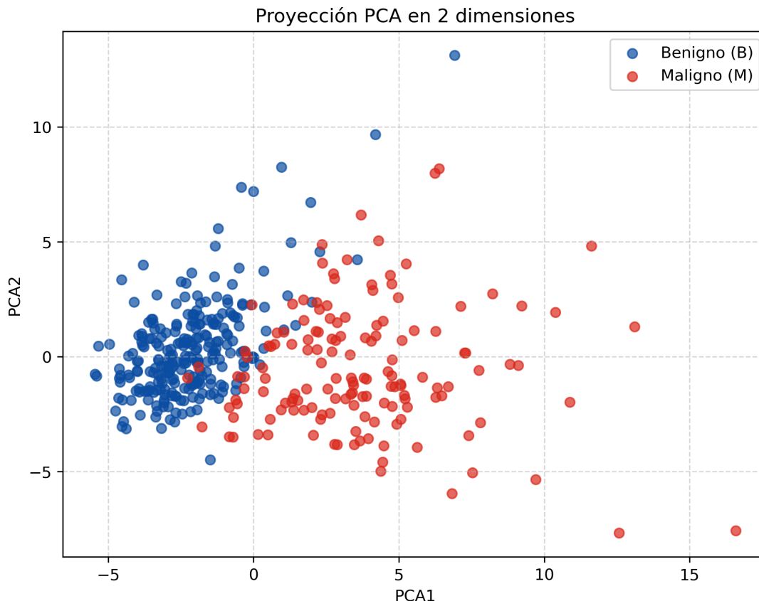
Figura 7: Proyección 2D de PCA sobre el conjunto de entrenamiento de Cancer. La separación entre clases es muy clara.
