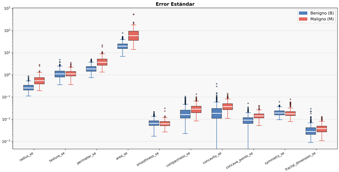
Figura 2: Boxplots comparativos del grupo de características se del conjunto Cancer. Escala logarítmica.
