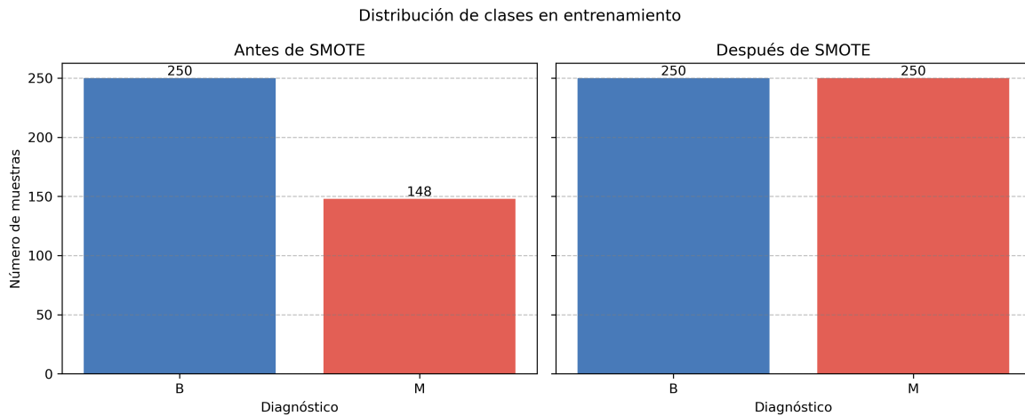
Figura 4: Distribución de clases en el conjunto de entrenamiento de Cancer, antes y después de aplicar SMOTE.
