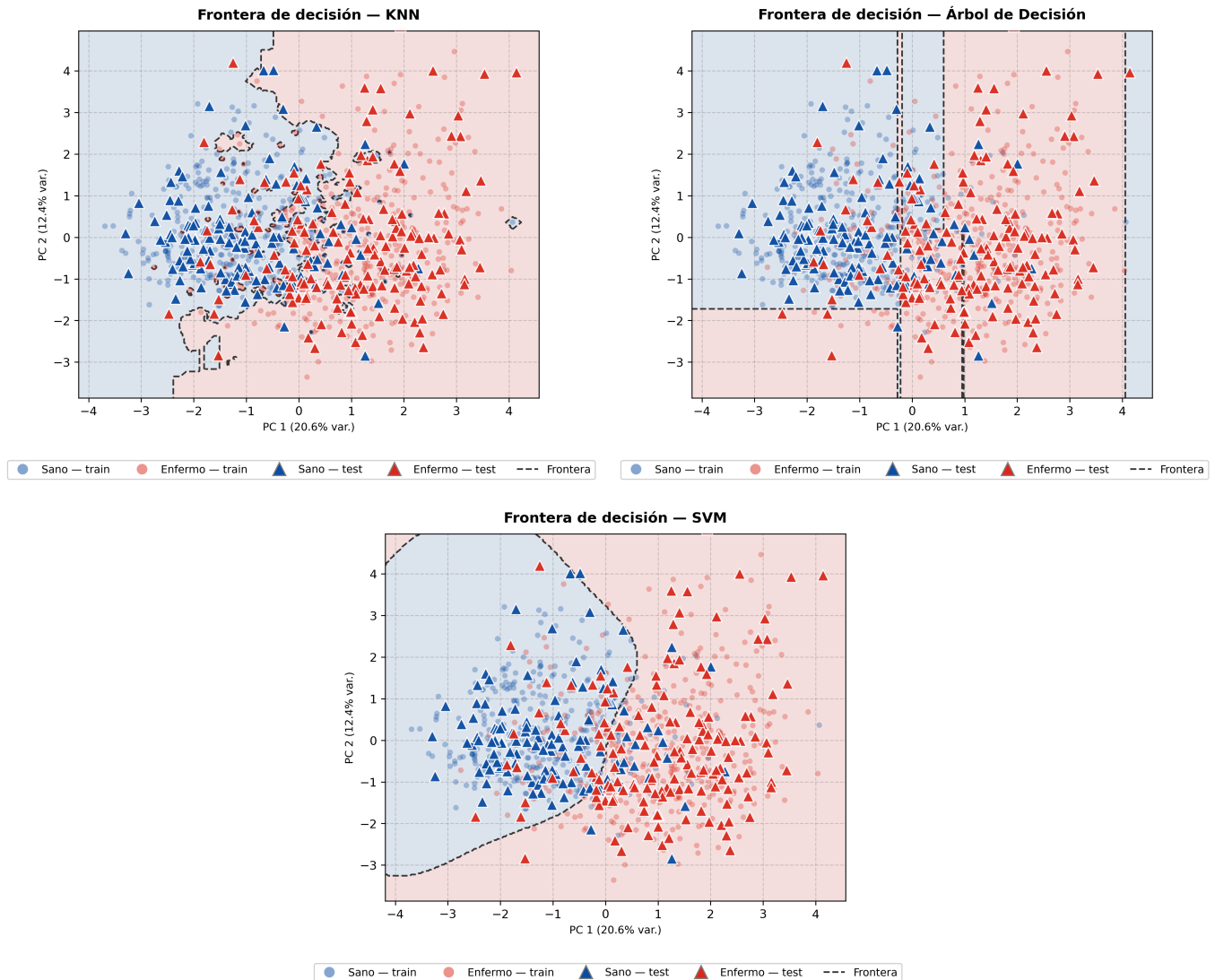
Figura 19: Fronteras de decisión en PCA 2D para Heart Disease: KNN (arriba izquierda), árbol (arriba derecha) y SVM-RBF (abajo).
