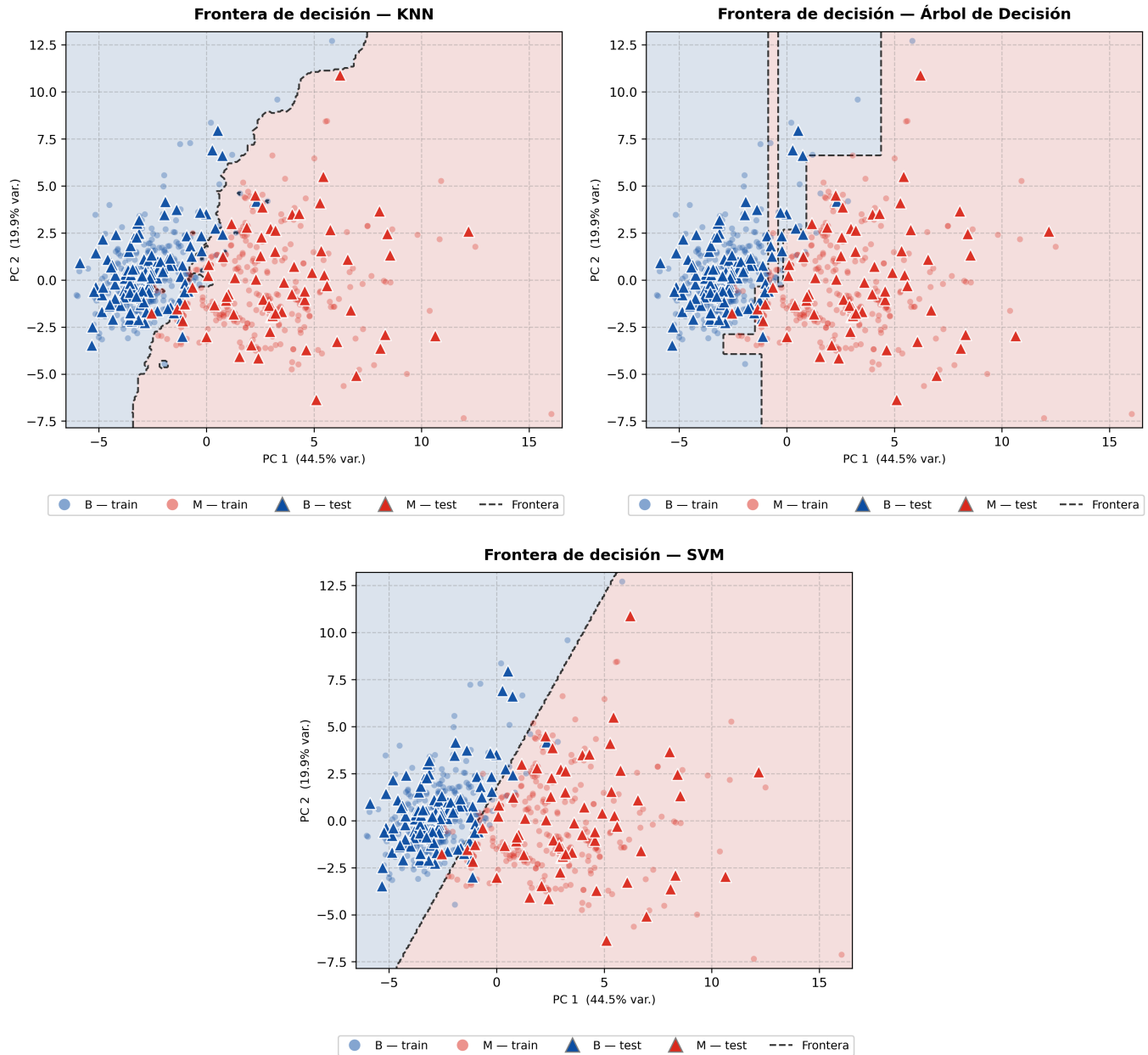
Figura 9: Fronteras de decisión en PCA 2D para Cancer: KNN (arriba izquierda), árbol (arriba derecha) y SVM lineal (abajo).
