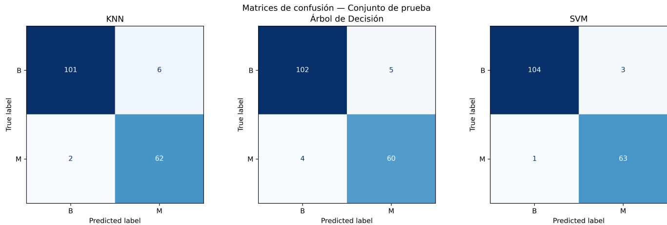
Figura 8: Matrices de confusión sobre el conjunto de prueba de Cancer para los tres modelos.
