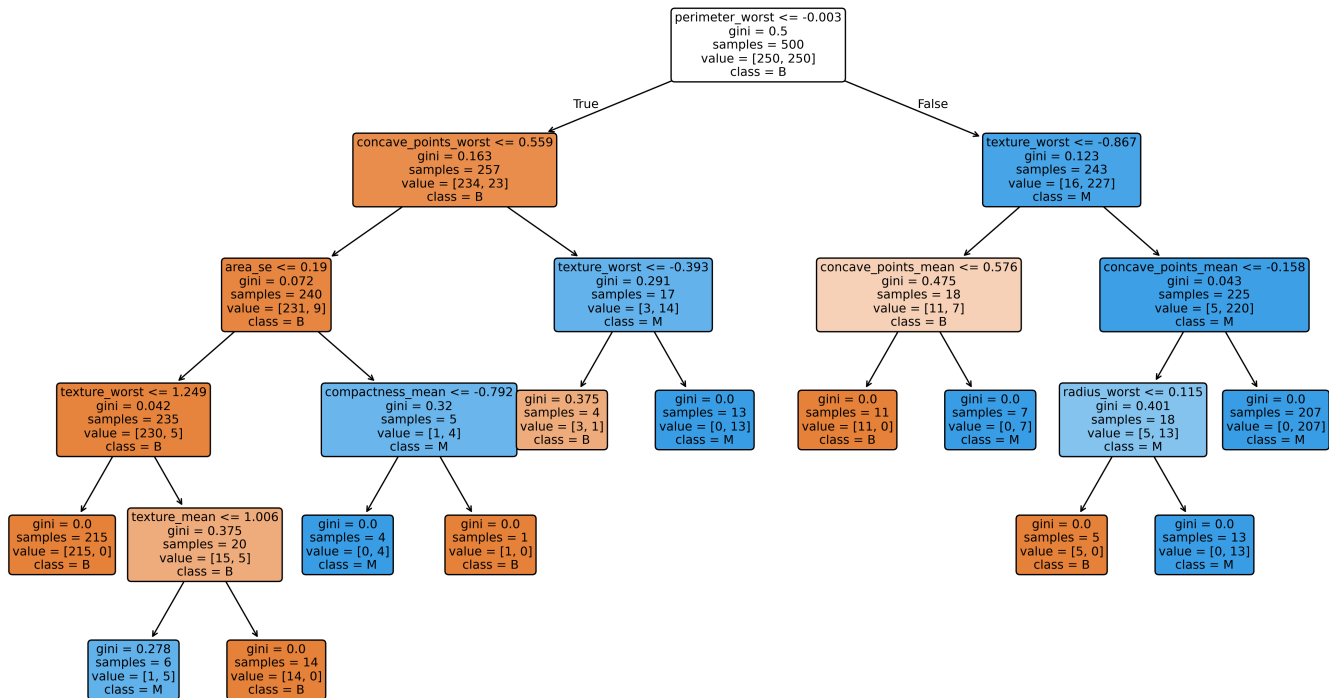
Figura 10: Árbol de decisión entrenado sobre Cancer con los mejores hiperparámetros.
