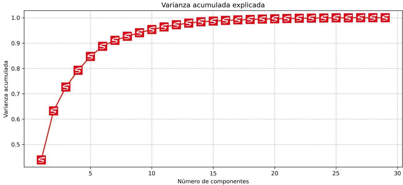
Figura 5: Varianza acumulada para PCA con Minka's MLE sobre Cancer. Los 29 componentes seleccionados absorben casi la totalidad de la varianza.
