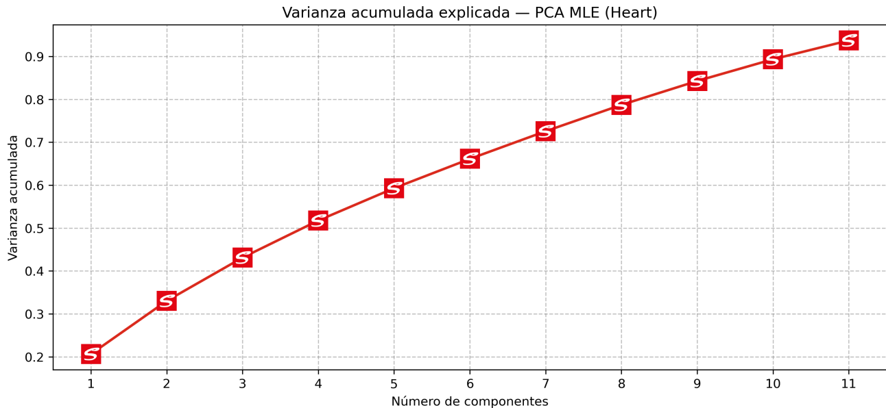
Figura 15: Varianza acumulada con PCA MLE sobre Heart Disease (11 componentes seleccionados).
