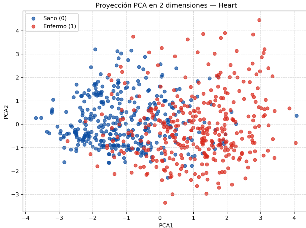
Figura 17: Proyección 2D de PCA sobre Heart Disease. El solapamiento entre Sano y Enfermo es considerable.
