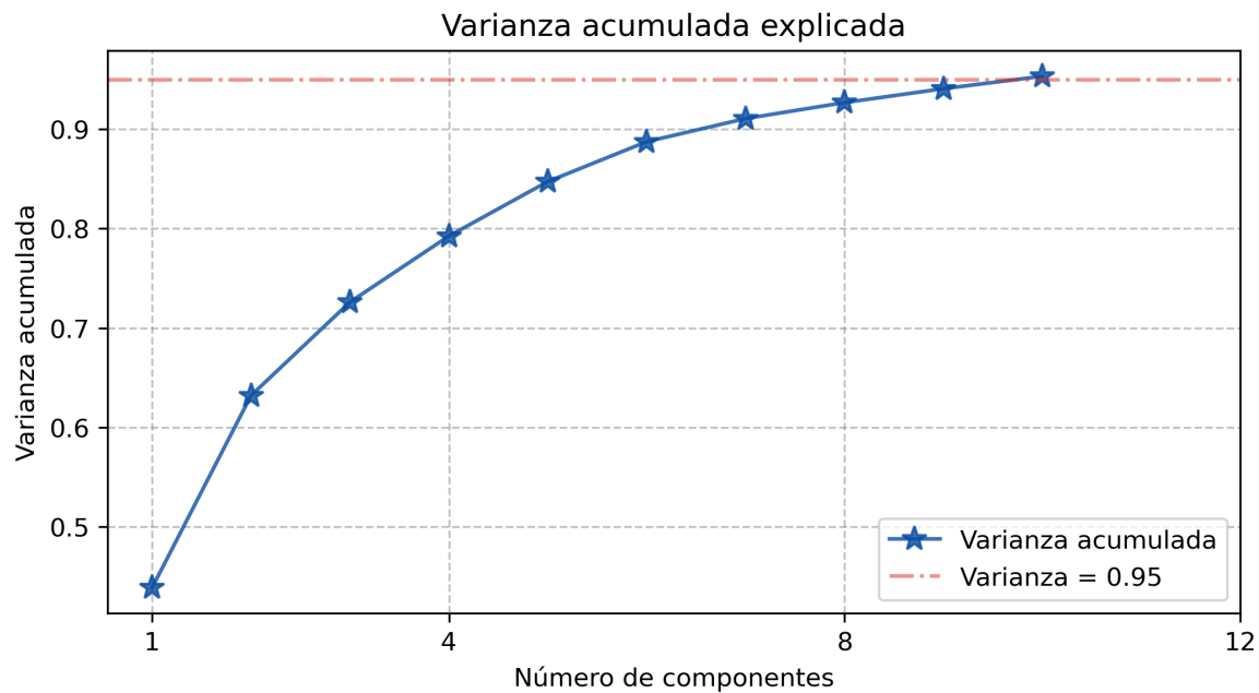
Figura 6: Varianza acumulada al fijar PCA con 95 %: bastan 10 componentes para superar el umbral.
