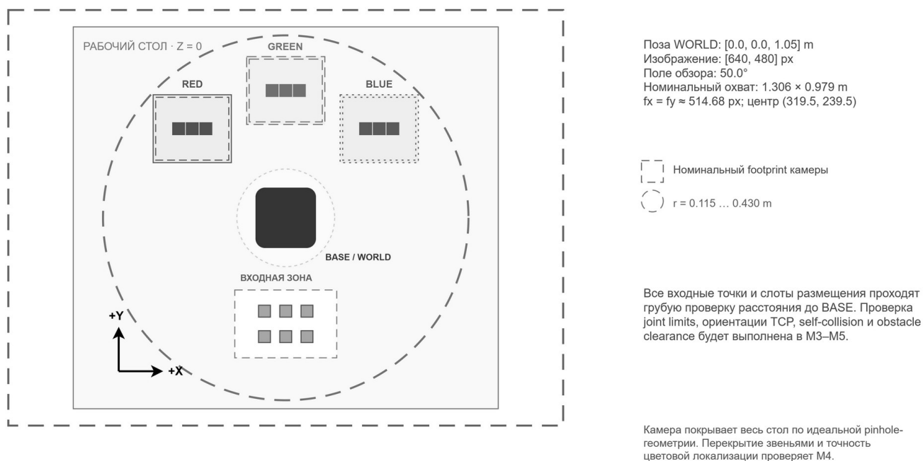
Рисунок 5.1 - Основная виртуальная камера и рабочие области; камера укладки placement_rgb описана отдельно
