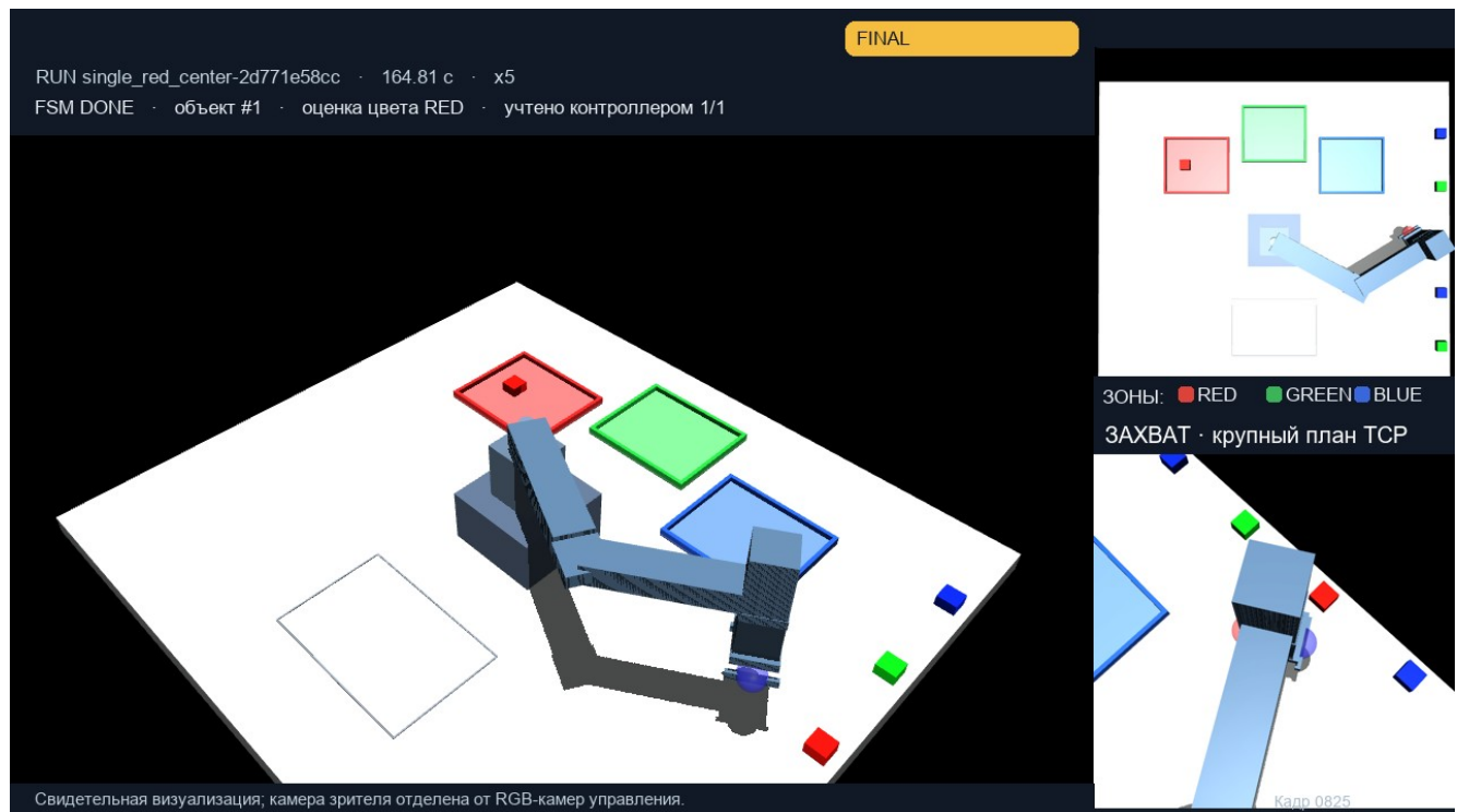
Рисунок 10.4 - Кадр завершенного виртуального цикла: вид сверху, состояние FSM и лоток RED
