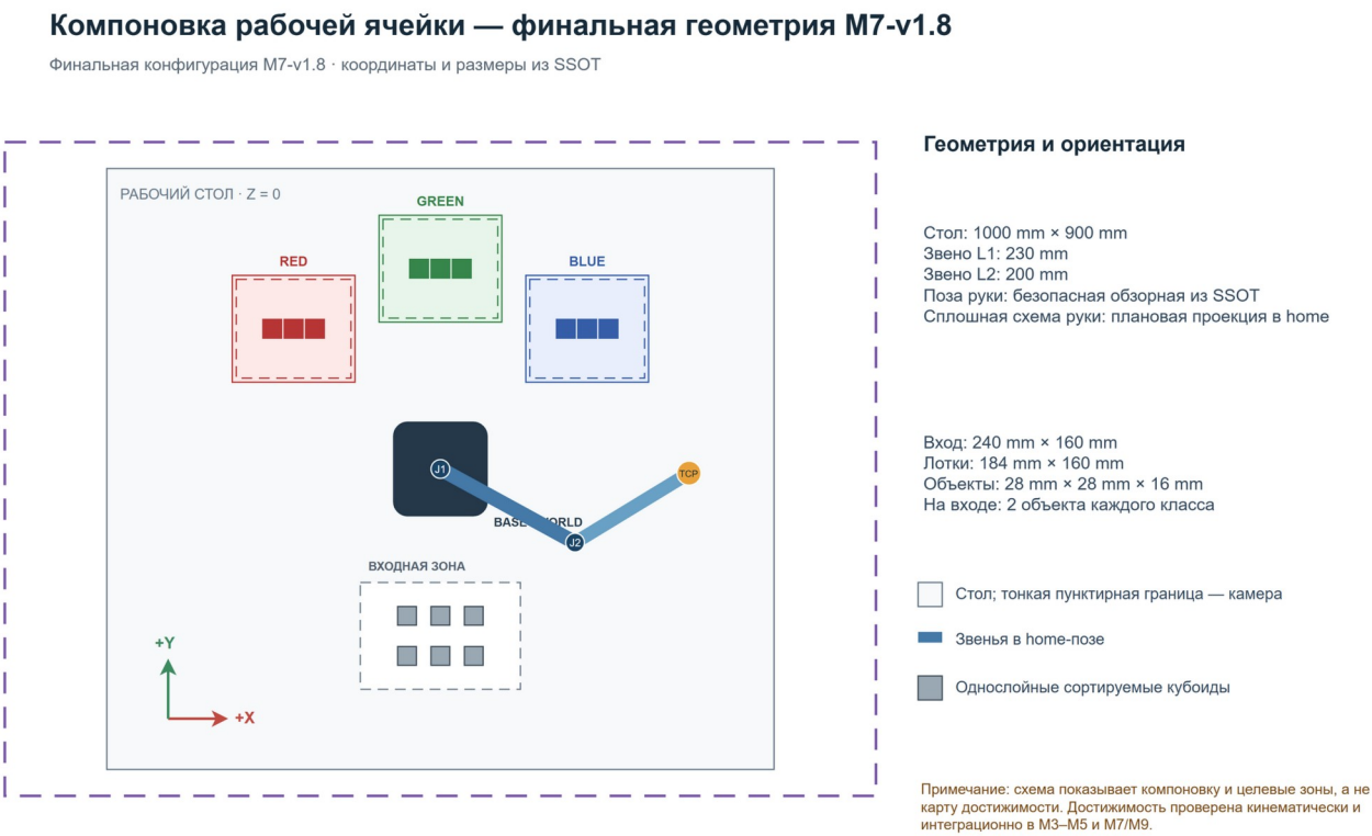
Рисунок 3.2 - Вид сверху: компоновка итоговой конфигурации M7-v1.8 из SSOT
