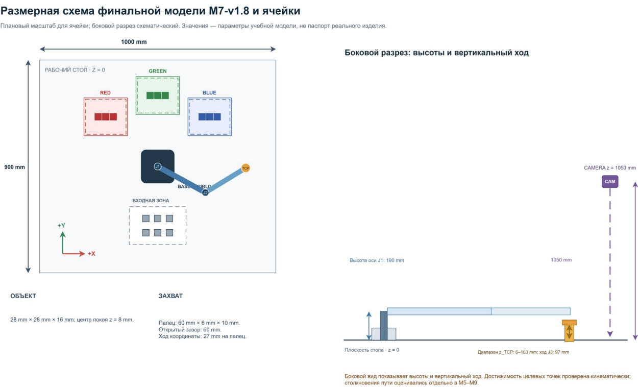
Рисунок 3.3 - Размерный вид итоговой ячейки: наружный размер лотка 184 × 160 mm
