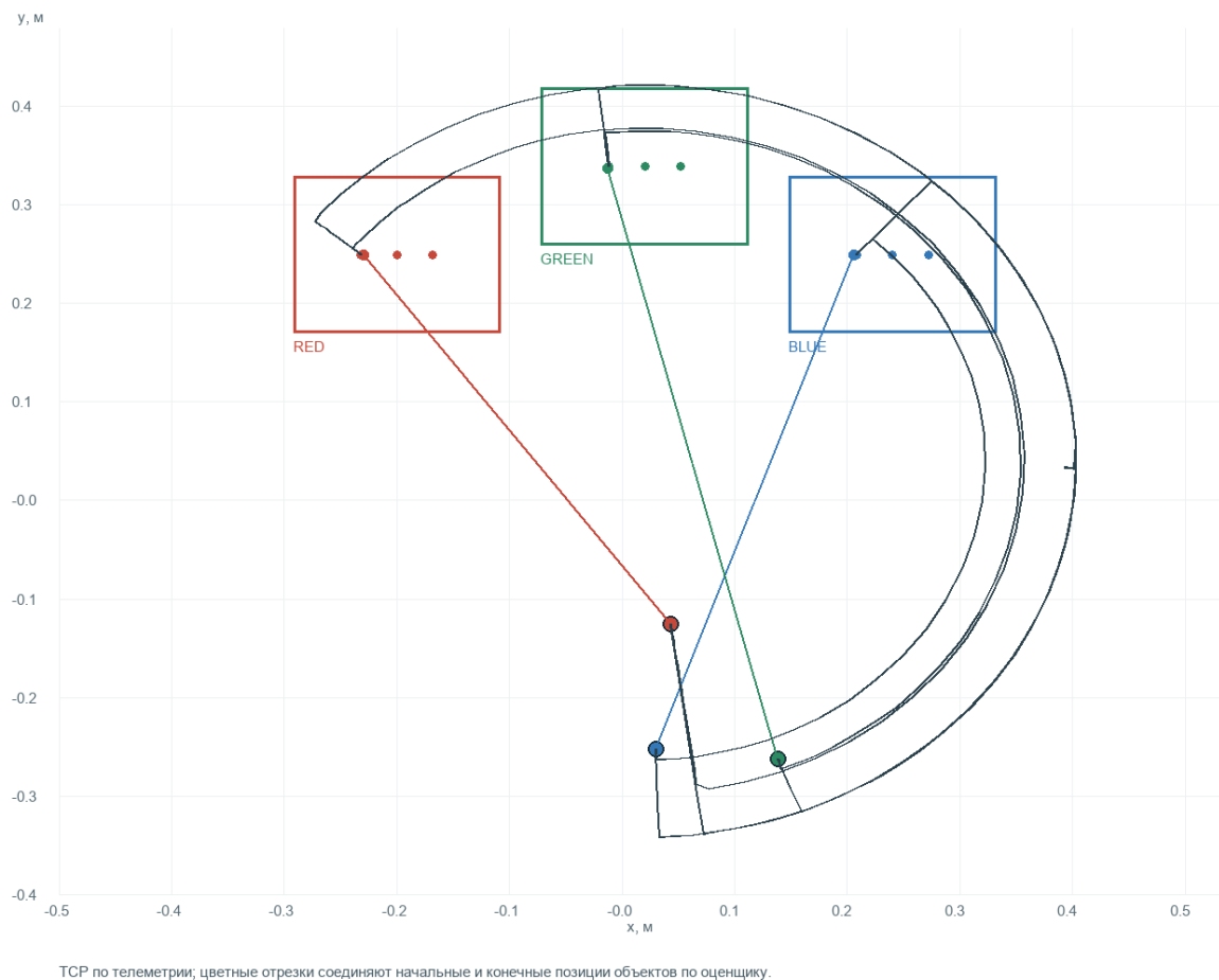
Рисунок 6.1 - Измеренная TCP-траектория полного успешного смешанного виртуального прогона М9
