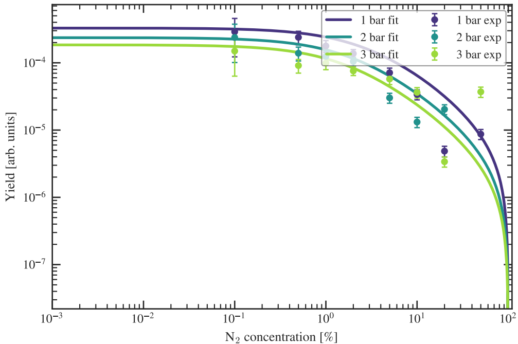
Ar--N 2 primary IR fit, 727 nm
