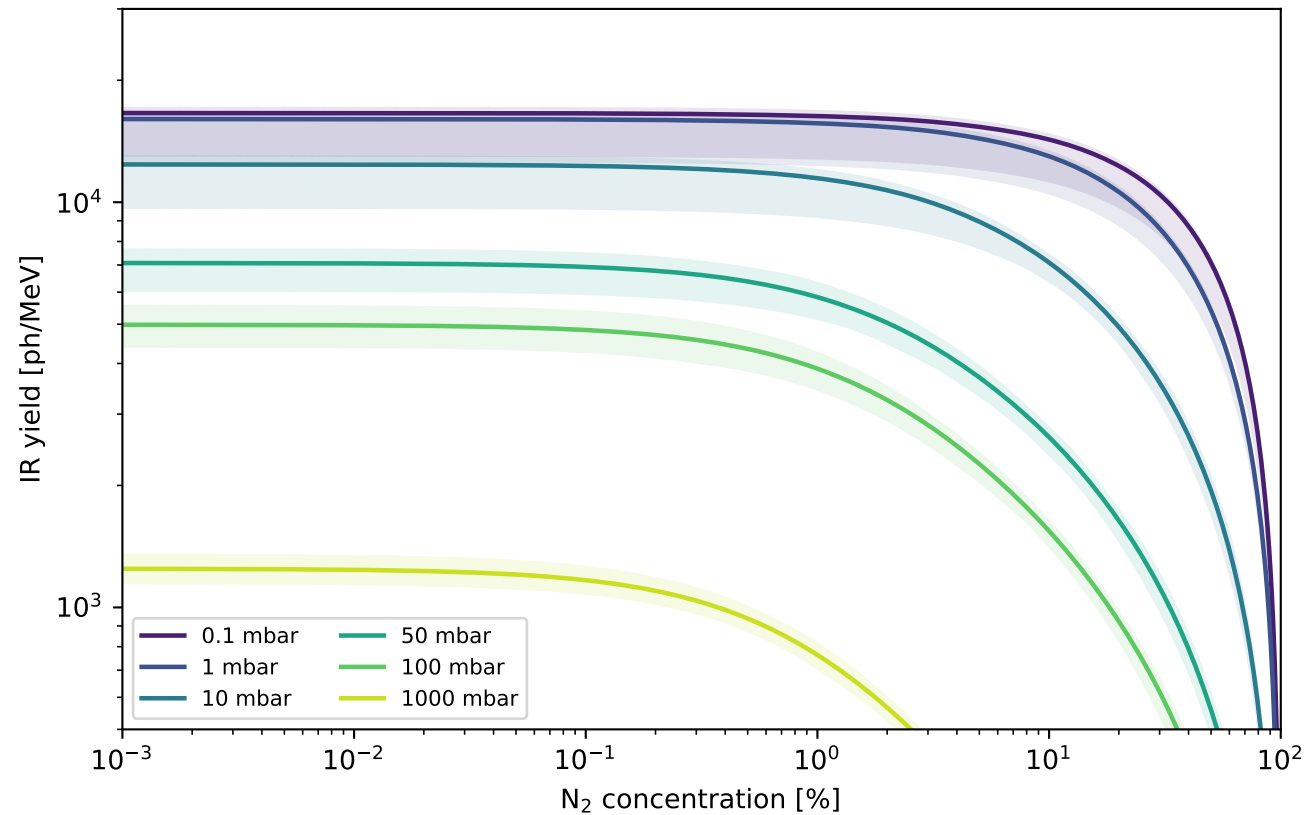
Ar--N 2 joint-fit IR prediction
