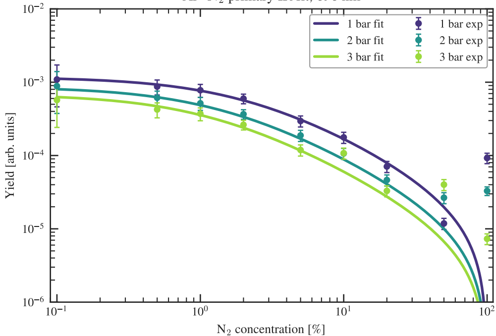
Ar--N 2 primary IR fit, 696 nm
