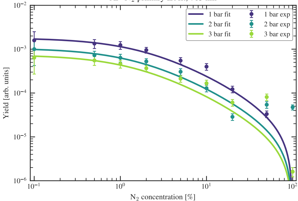
Ar--N 2 primary IR fit, 763 nm
