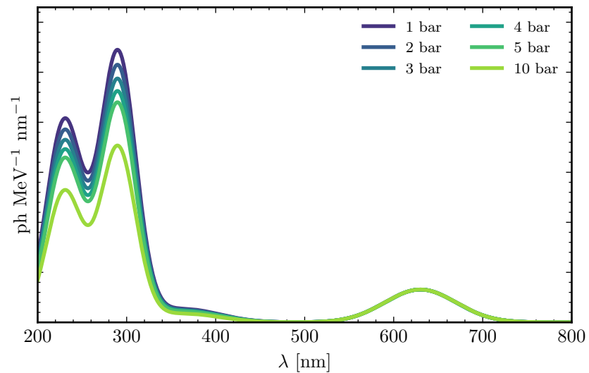
Ar-CF 4 , 100% CF 4
