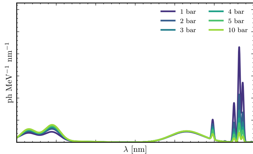
Ar-CF 4 , 100% CF 4
