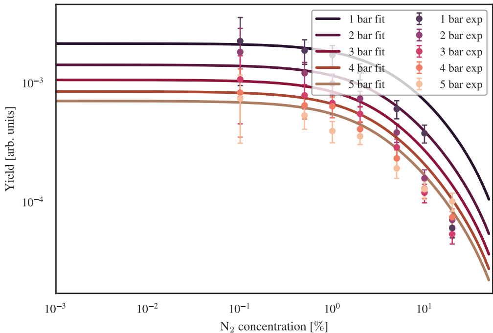
Ar--N 2 primary IR fit, 772 nm
