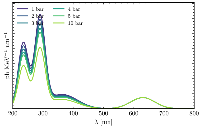
Ar-CF 4 , 100% CF 4
