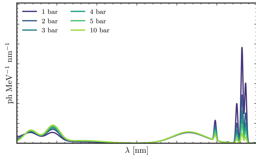
Ar-CF 4 , 100% CF 4
