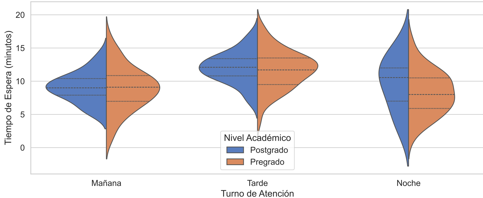
Distribución del Tiempo de Espera por Turno y Nivel Académico
