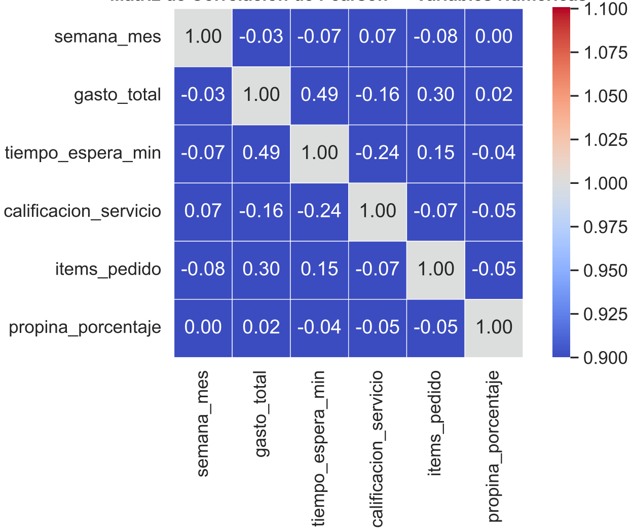
Matriz de Correlación de Pearson — Variables Numéricas
