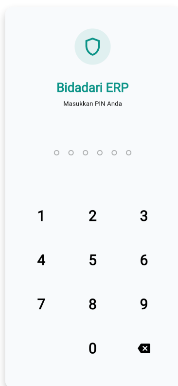
Halaman Login
