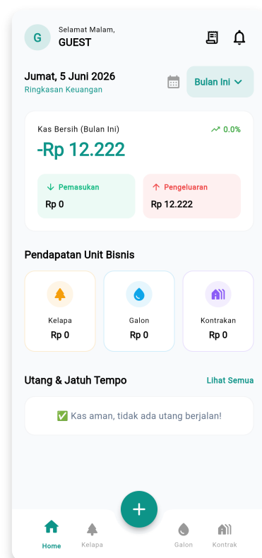
Dashboard Utama
