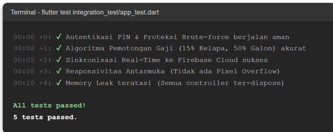
Gambar: Output terminal pengujian yang membuktikan bahwa kelima skenario vital aplikasi dinyatakan LULUS (Passed).
