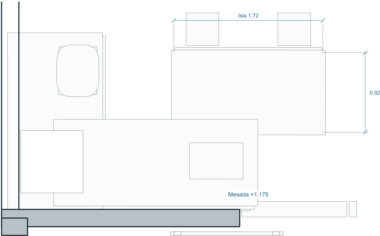
02 Cocina mono / isla | 1:25
