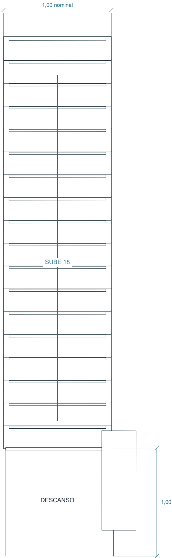
01 Planta / acceso | 1:20
