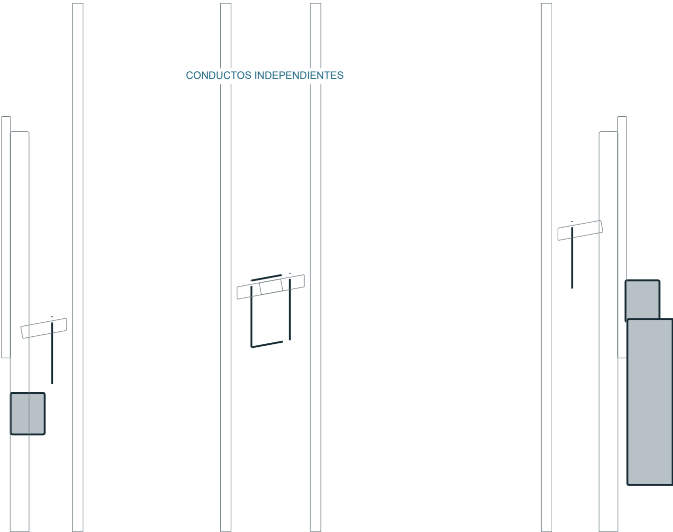
D07 Paso de conductos / X=21,50 | 1:5
