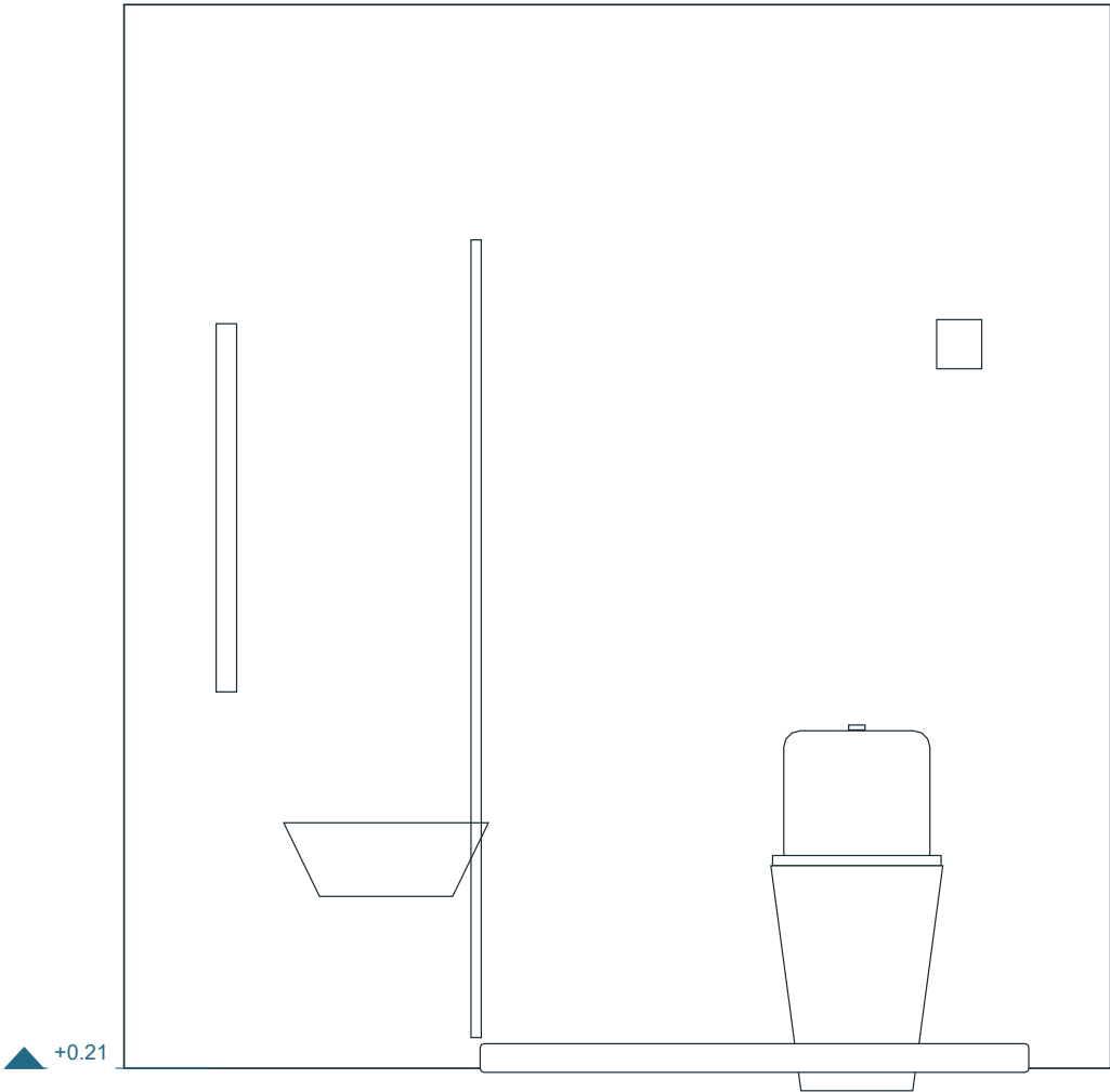
Elevacion interior / artefactos | 1:20
