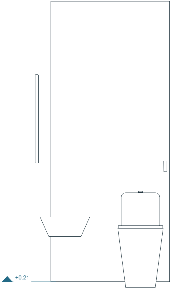
Elevacion interior / artefactos | 1:20
