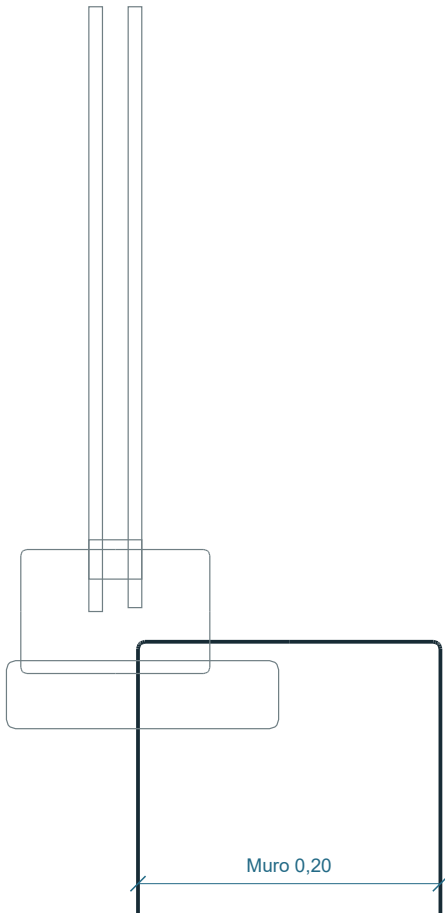
D06 DVH / antepecho / Z=3,00 | 1:5
