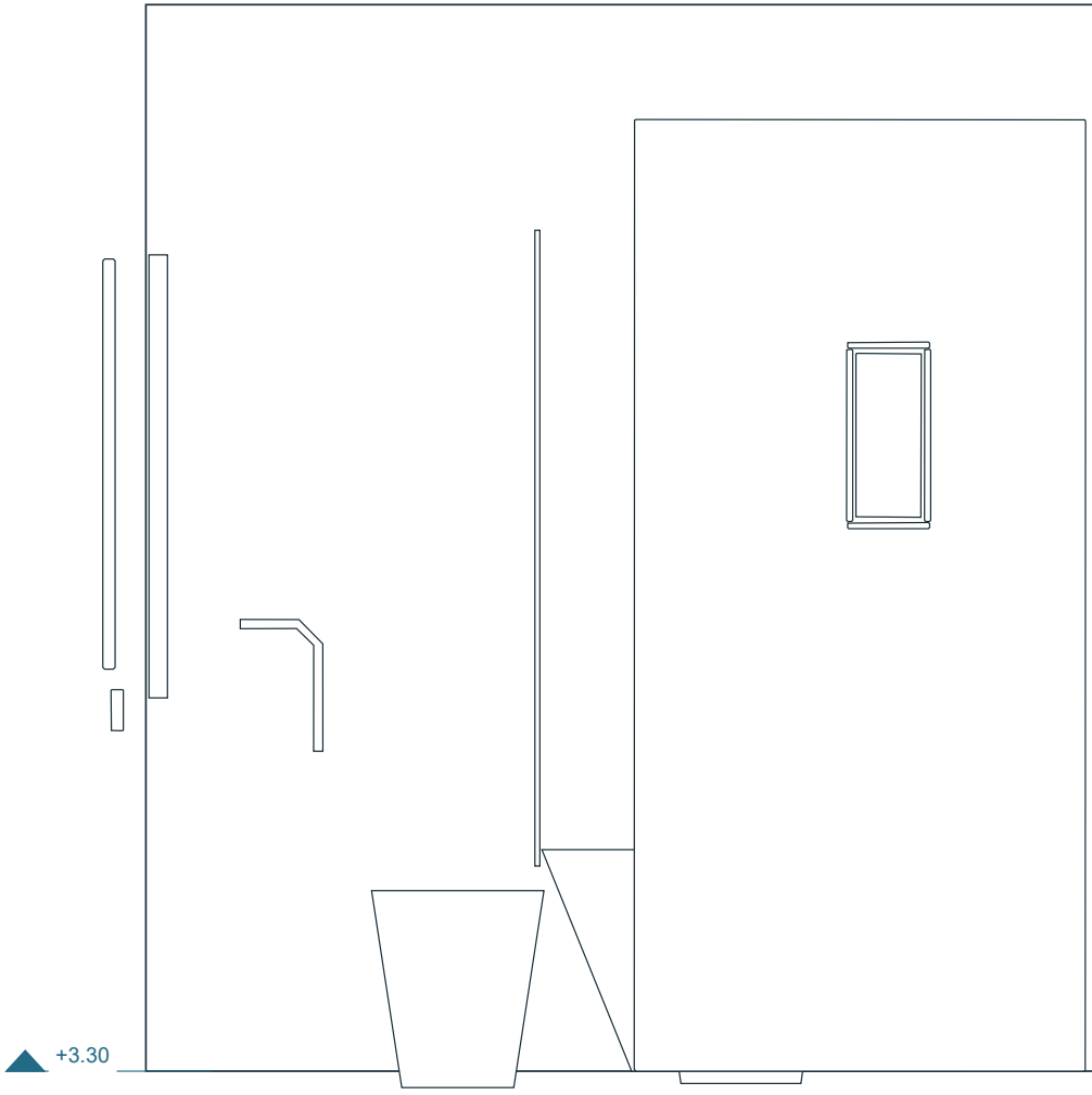
Elevacion interior / artefactos | 1:20
