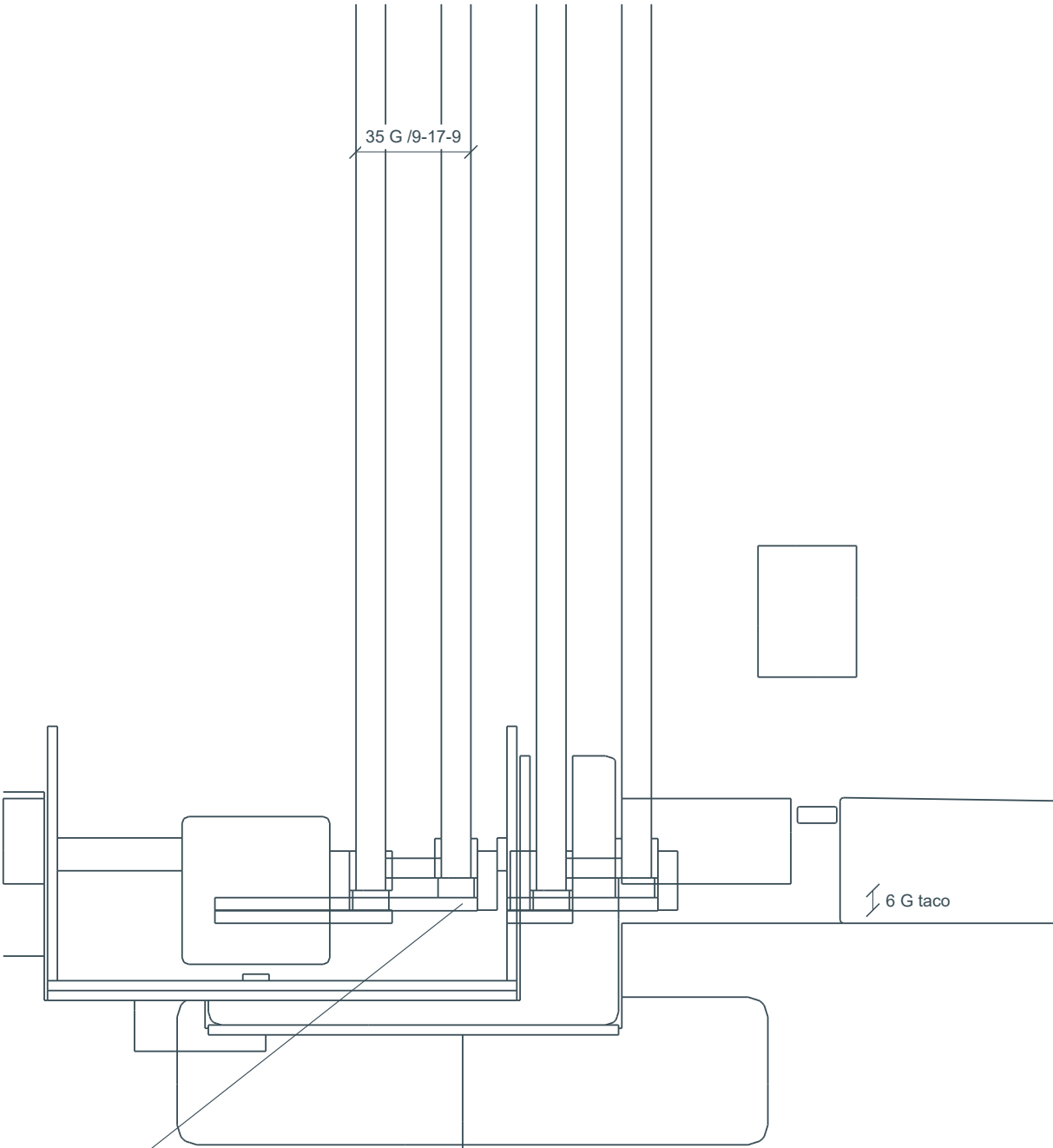
21 Acristalamiento / corte por tacos | 1:2
