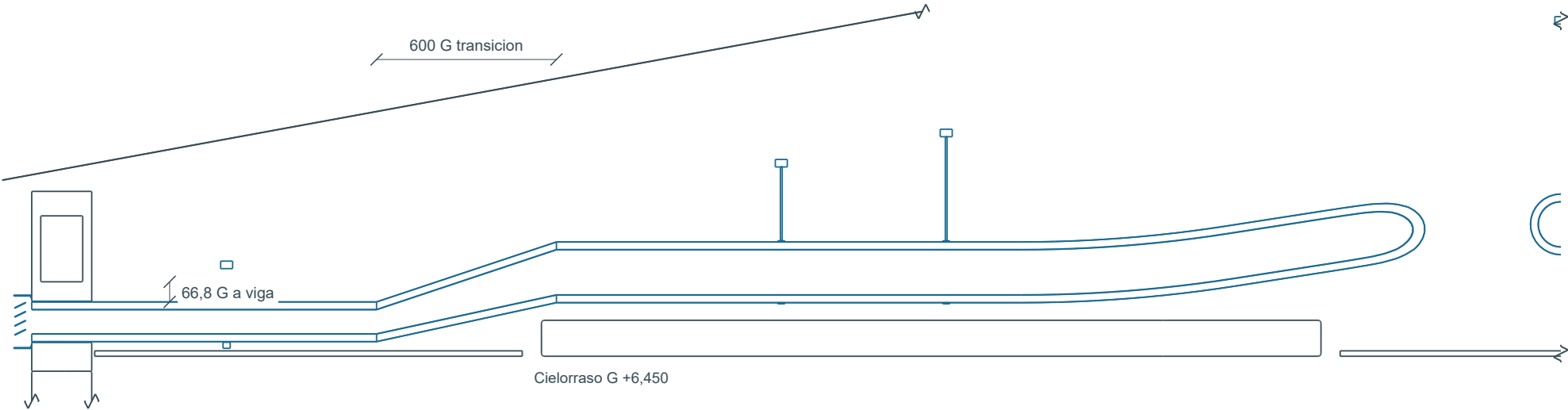
20 Frente / corte X17,64 | 1:20
