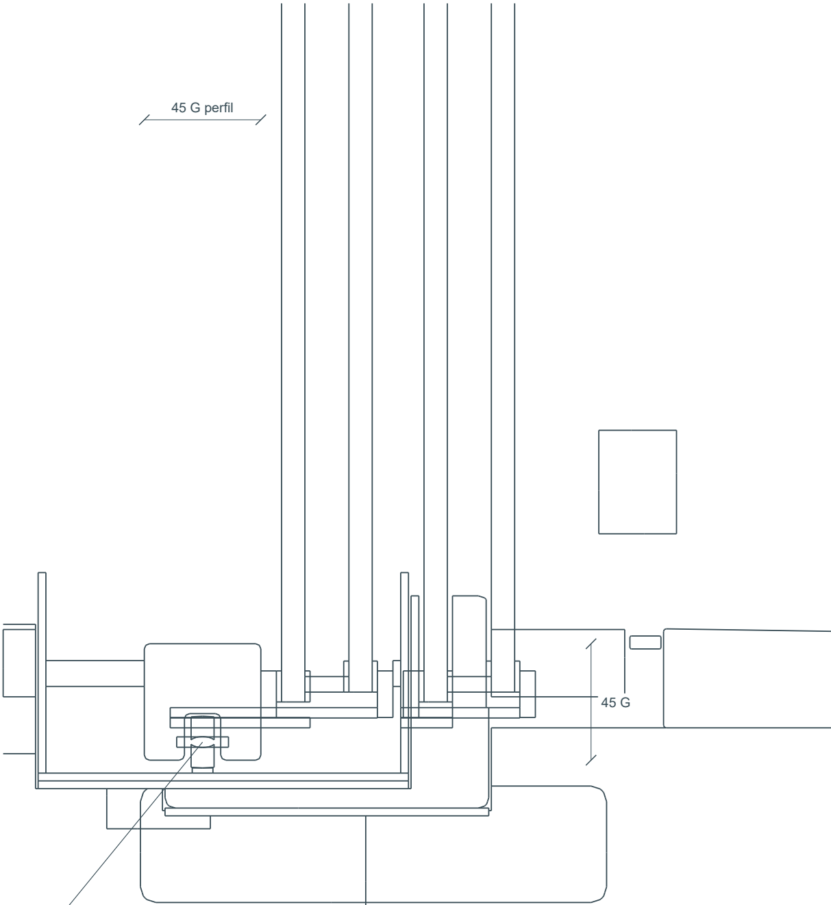
20 Rodadura / corte exacto de la geometria | 1:2
