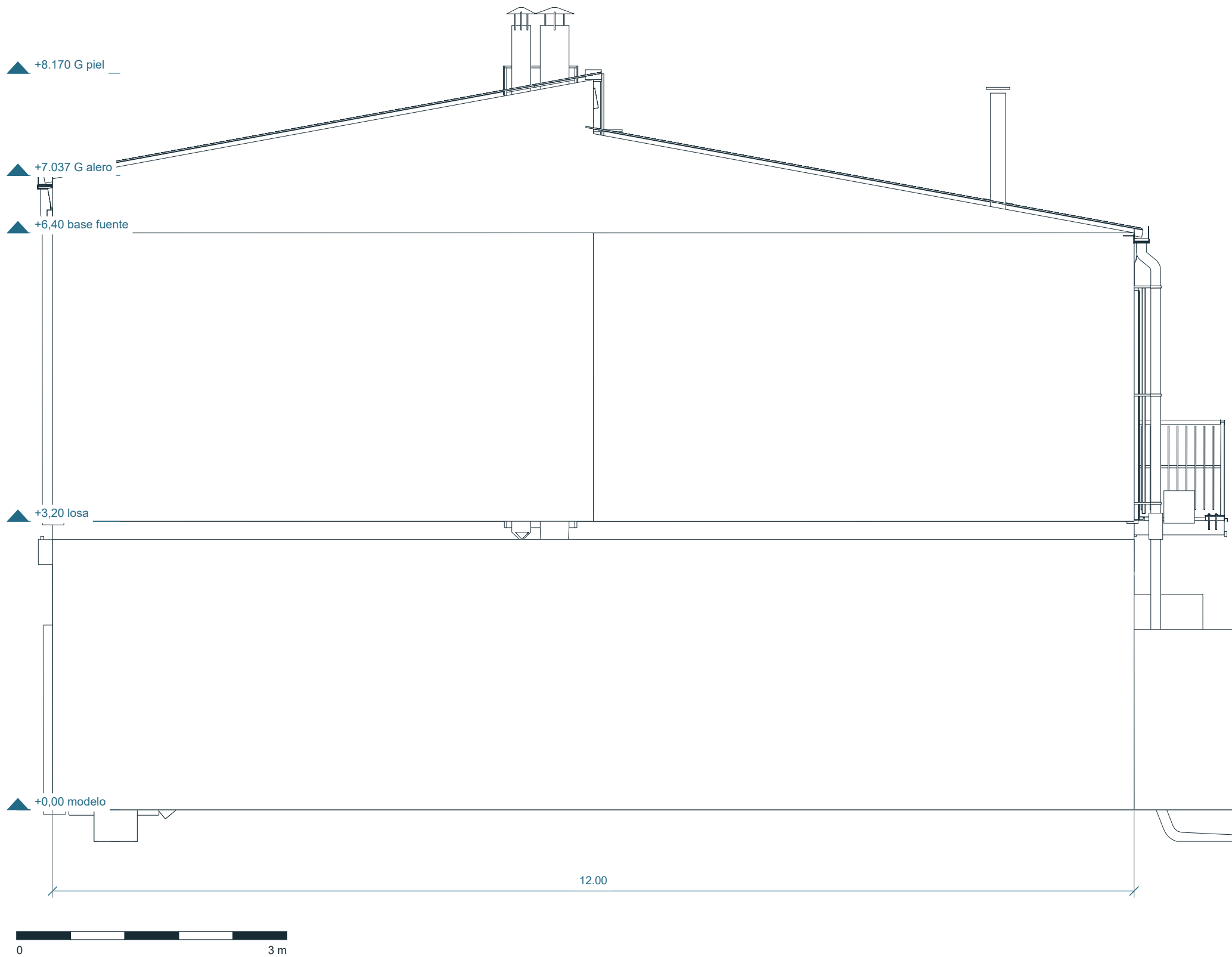
04 Medianera lateral | 1:50
