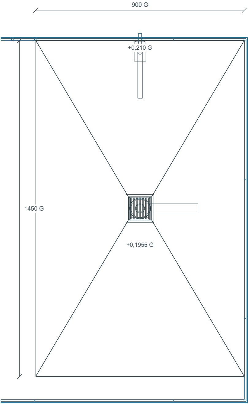
24 Ducha PB / planta | 1:10
