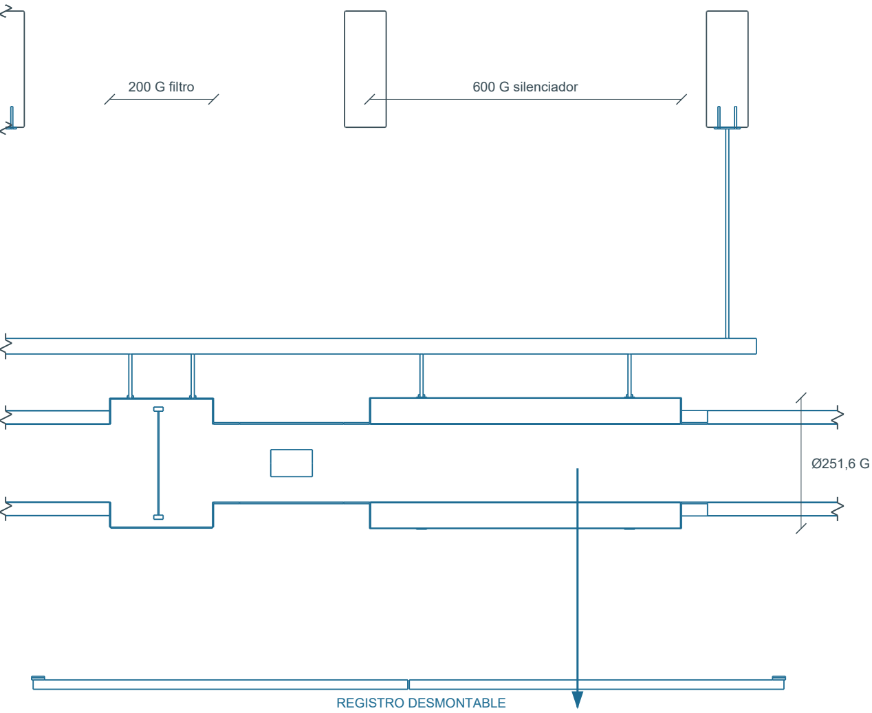
18 Equipo / corte Z4,68 | 1:10
