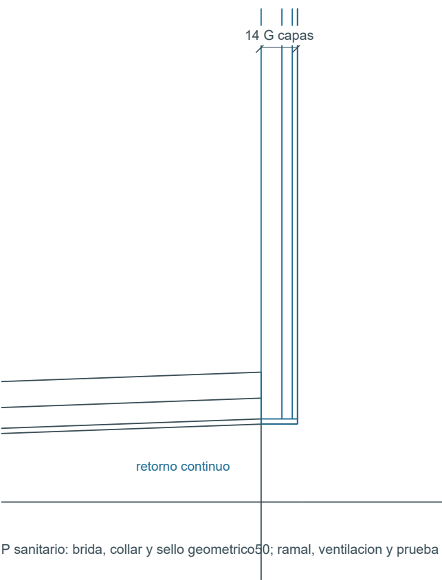
27 Piso-muro PB / Z1,40 | 1:2
