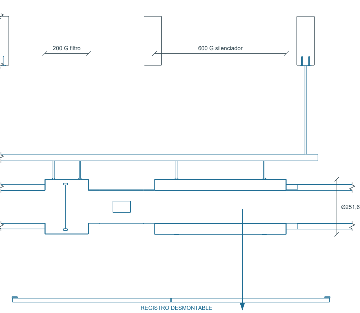
18 Equipo / corte Z4,68 | 1:10
