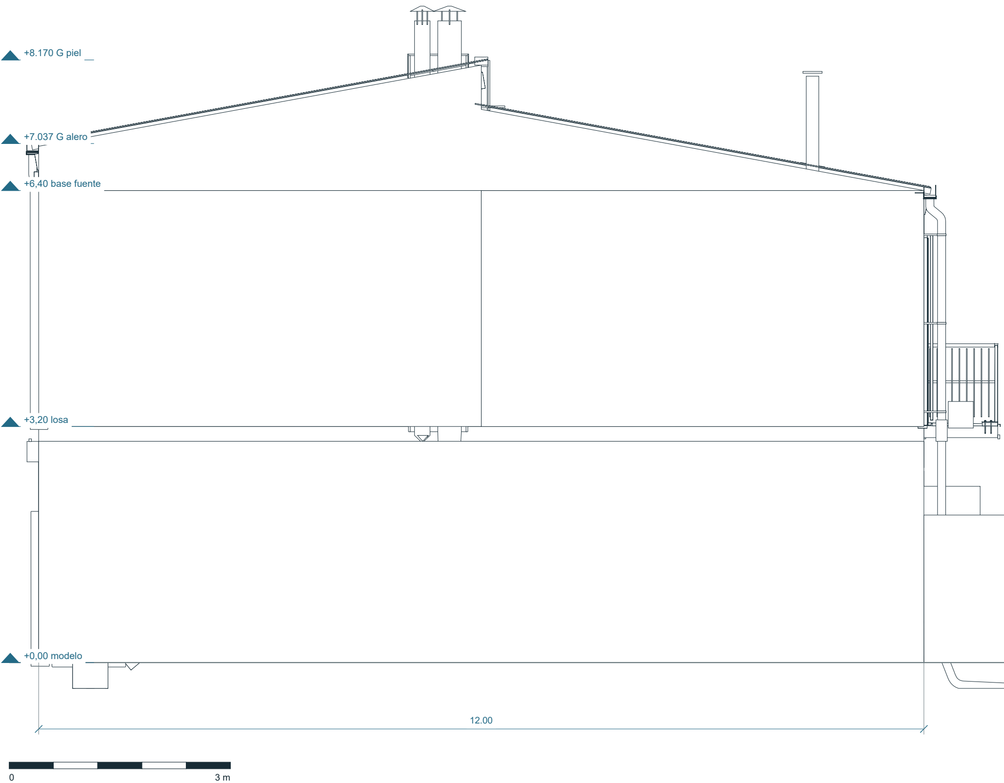
04 Medianera lateral | 1:50
