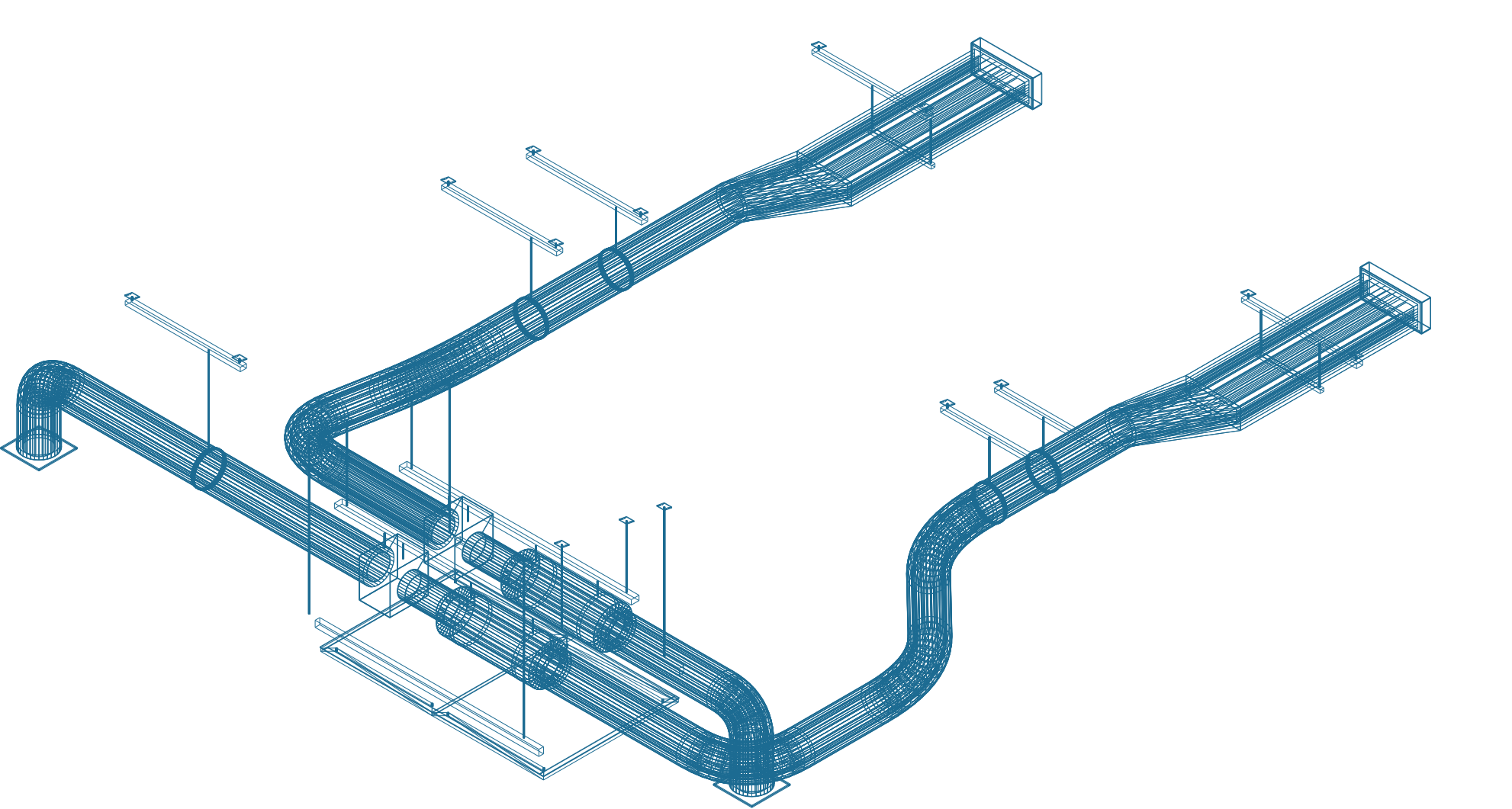
17 Axonometria de montaje / sin escala
