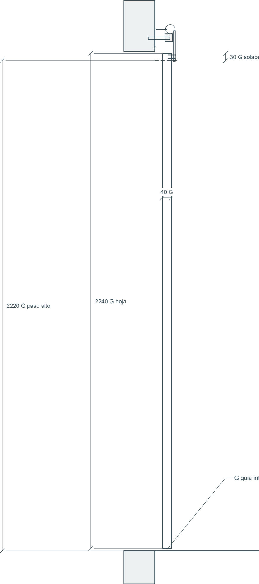
19 Corredera modelada / vista parcial G | 1:10
