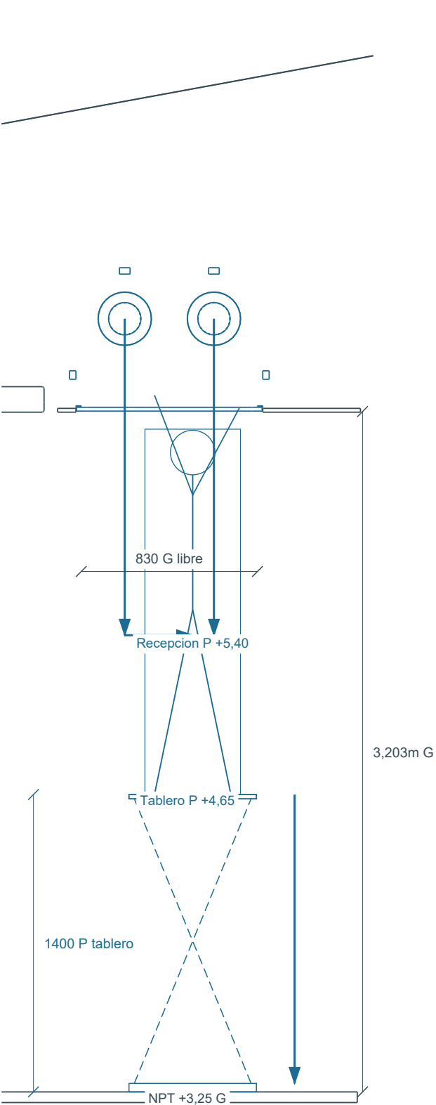
19 Acceso / X19,40 + P | 1:25
