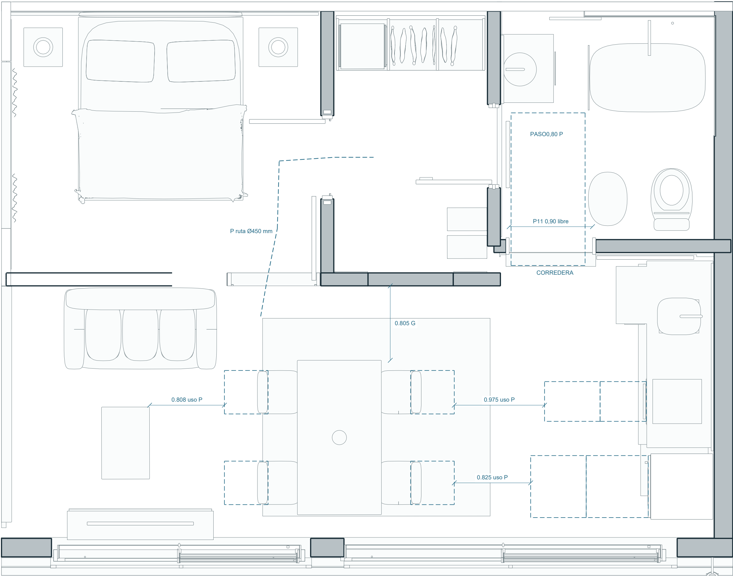
01 Vivienda / accesos, mobiliario y huellas de uso | 1:25
