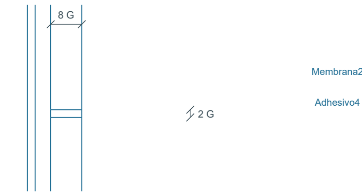
24a Junta pasante / X21,35 | 1:1
