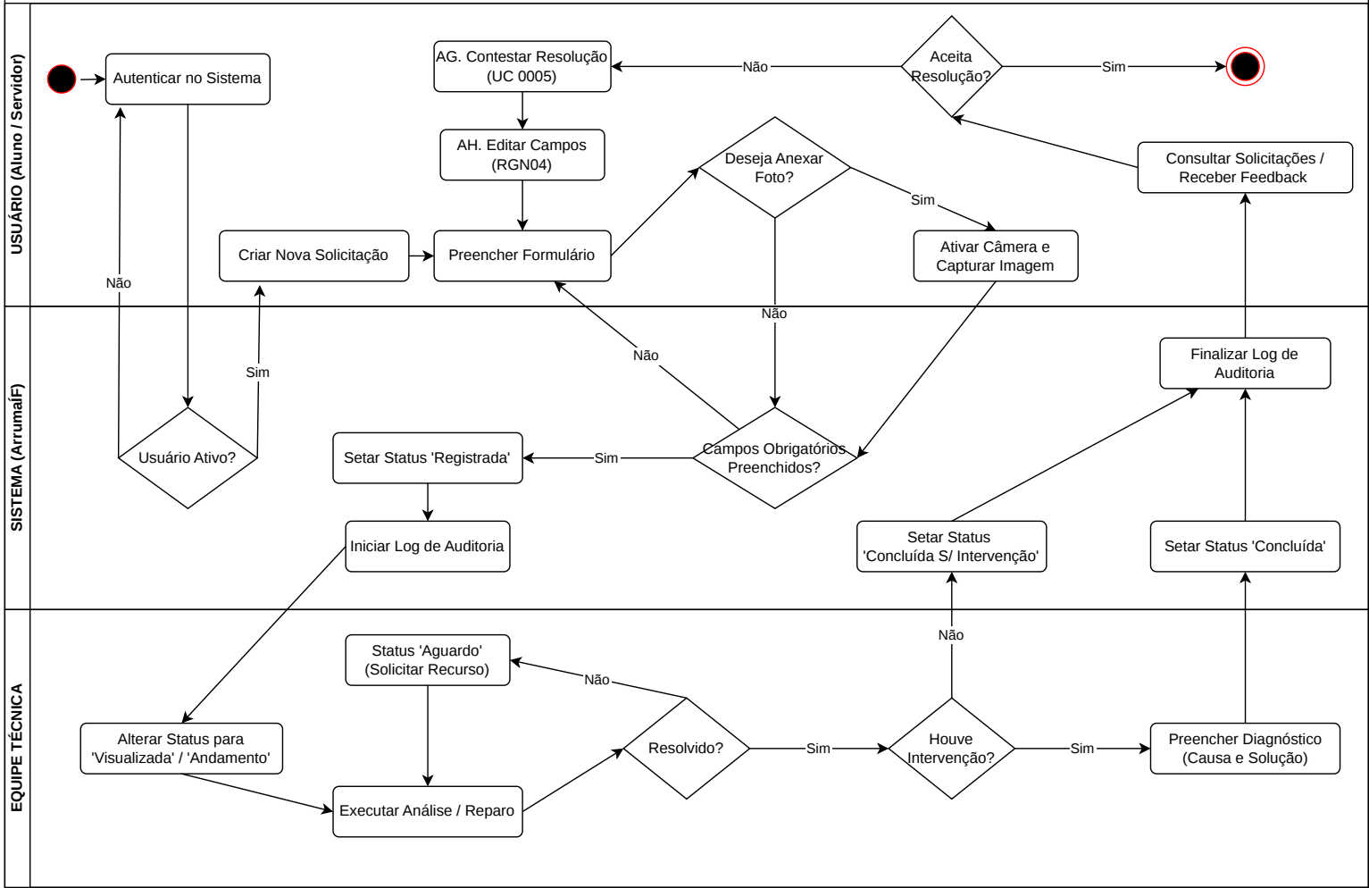
Diagrama de Atividades - ArrumalF
