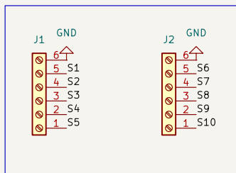
Signal Jst
