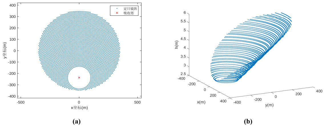
图9 调节后定日镜场中定日镜排布图
