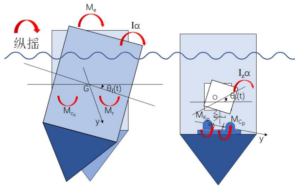
图 10 纵摇运动受力分析示意图
