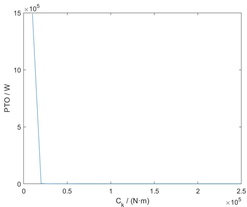
图 17 扭转弹簧刚度的稳定性分析图
