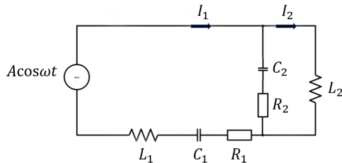
图 6 力电比拟等效电路图
