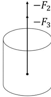
图3 振子受力分析图
