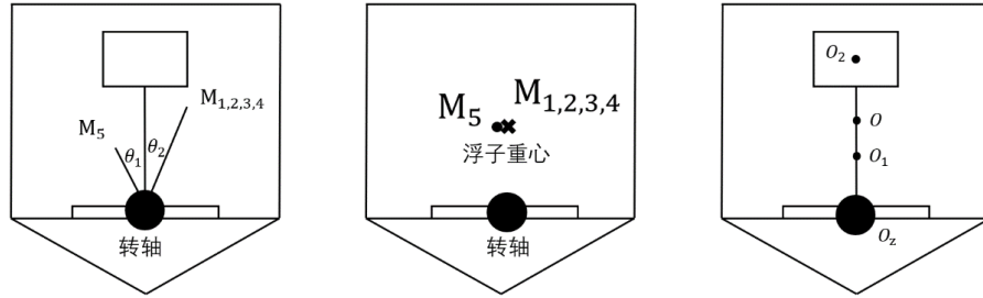
图9 浮子力矩分析示意图
