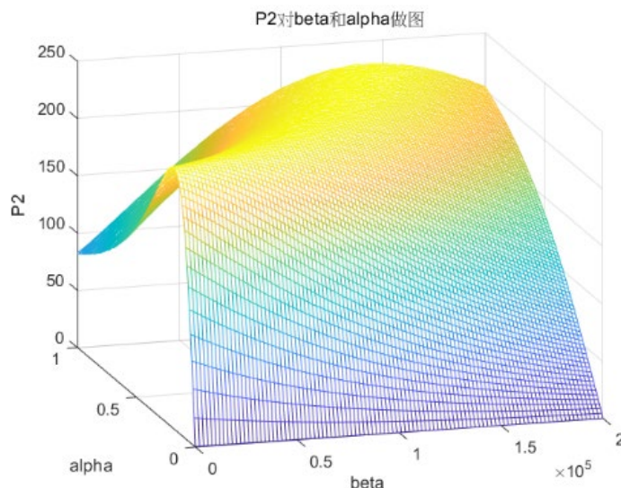
图 8 P 对 \beta 和 \alpha 作图
