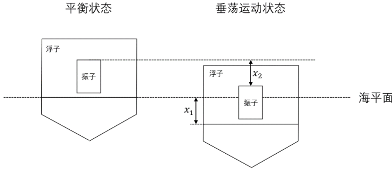
图 1 浮子坐标示意图
