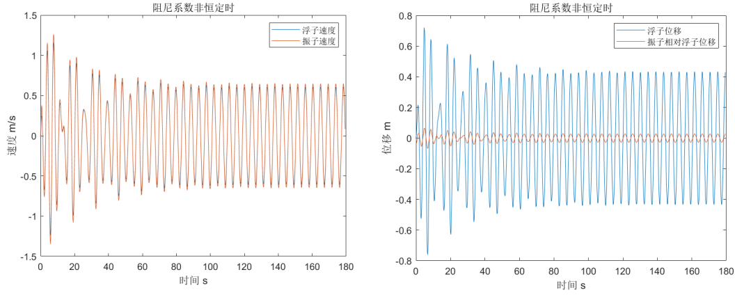
图 5 阻尼系数非恒定时结果曲线
