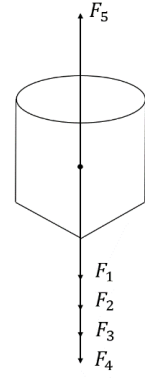
图 2 浮子受力分析图
