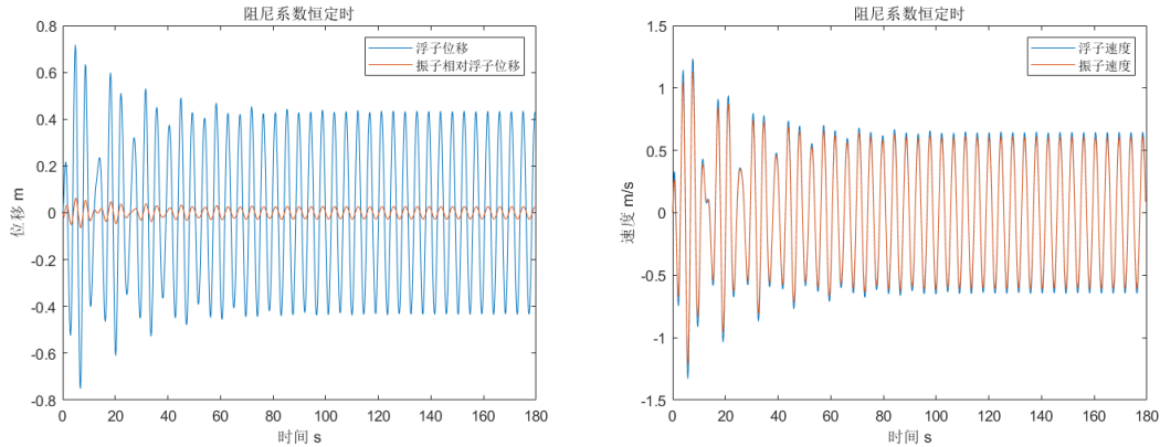
图4 阻尼系数恒定时结果曲线
