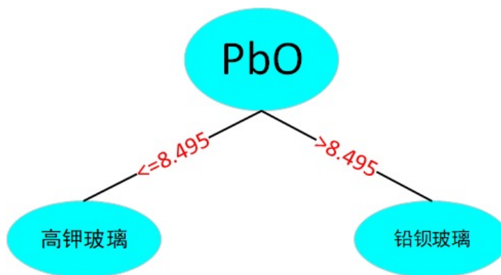
图 4 未风化类型决策树
