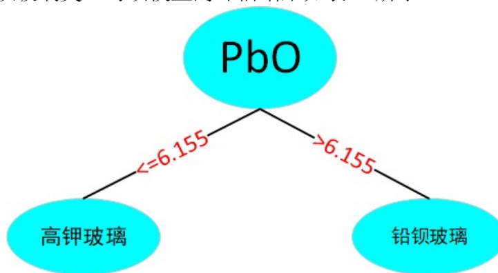
图 5 未风化类型决策树
