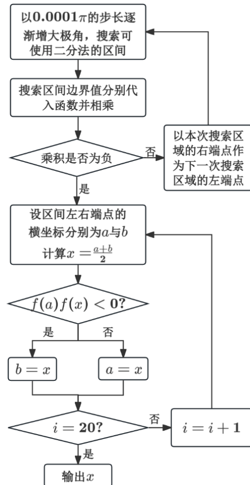
图 7 二分法求解龙头前把手位置流程图
