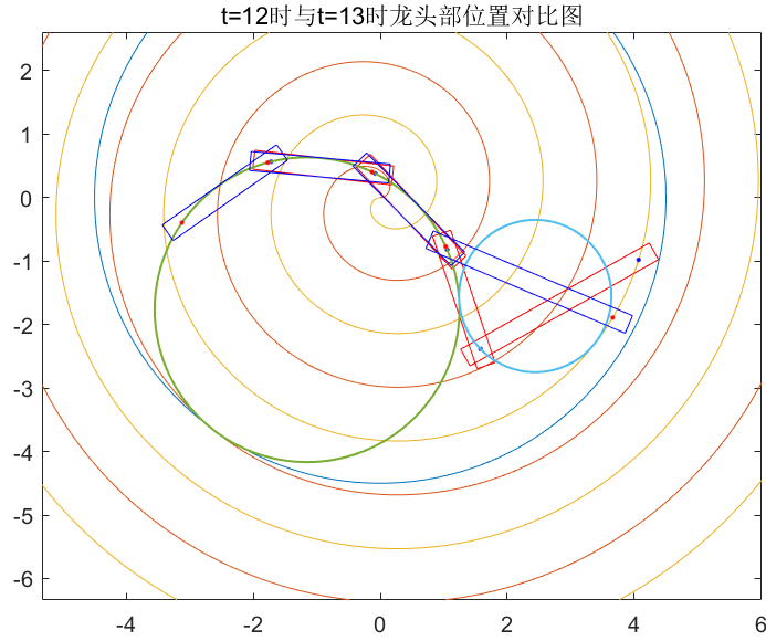
图 27 第 12 s~13 s 龙头部分的轨迹图
