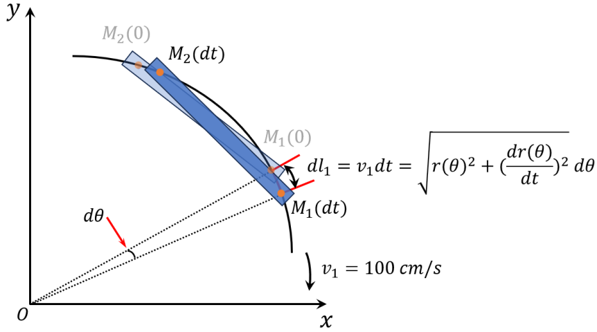
图3 螺旋线弧长的积分求解
