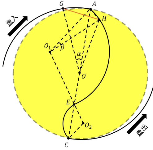
图 4.20: 情况二示意图
