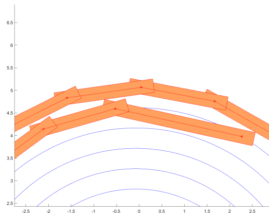
图 4.15: 最小螺距下最接近碰撞时刻示意图（放大）
