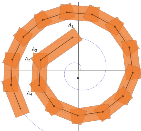
图 2.6: 板凳龙盘入示意图（橙色矩形为板凳）
