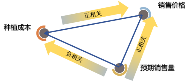
图 7 相关性分析
