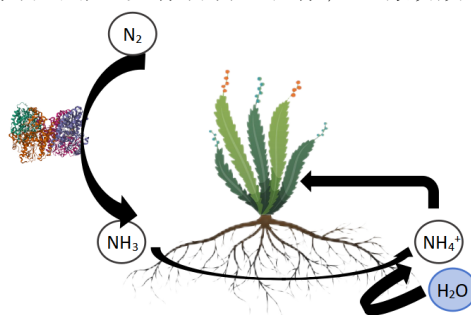
图 1 固氮原理
