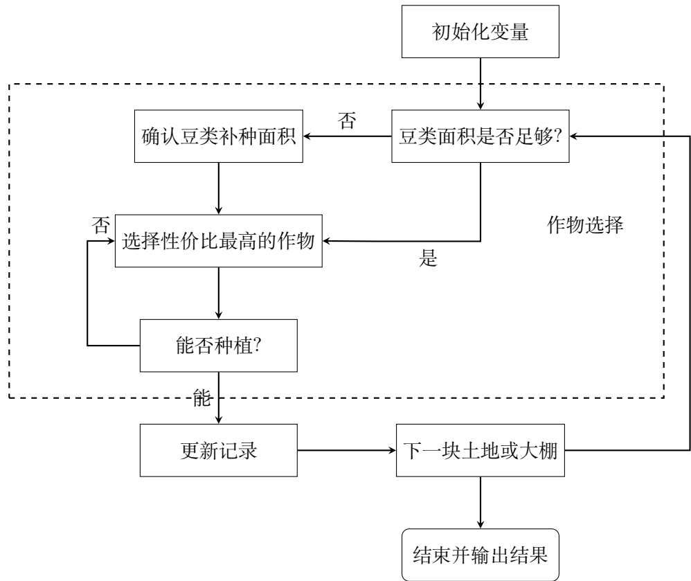
图 5 贪心策略
