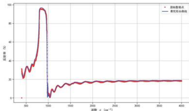
图 6: 反演参数曲线与真实碳化硅 10 度入射角反射率曲线的匹配情况
