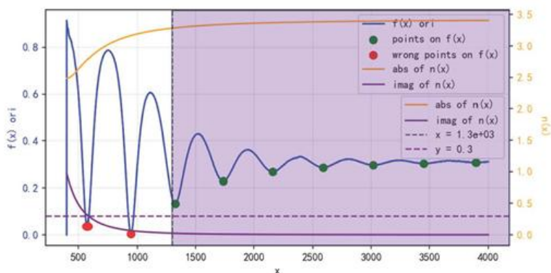
图 13: 附件 3 直接求解数据点对应的的外延层吸收率情况
