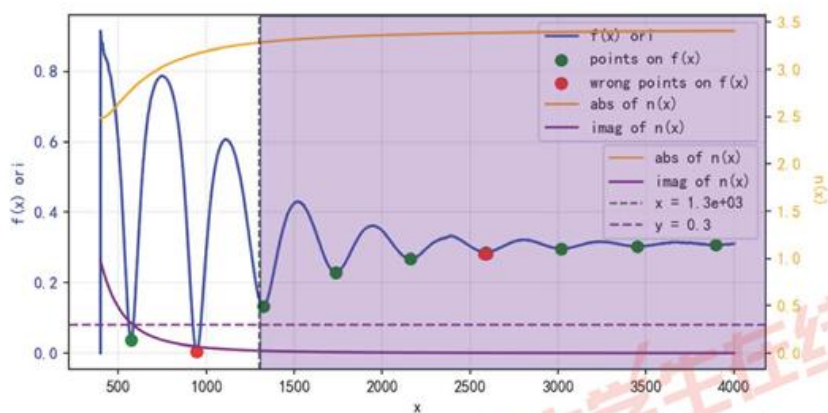
图 14: 附件 4 直接求解数据点对应的的外延层吸收率情况
