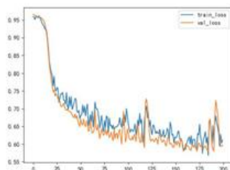
图 17 模型训练损失
