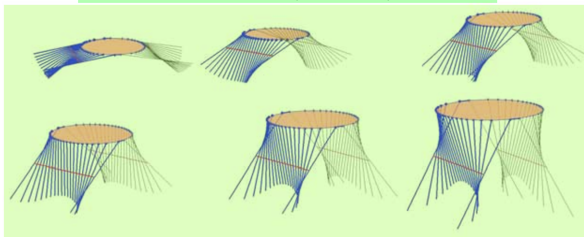
图 5-7 长方形木板到桌子的动态变化过程
