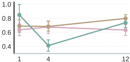
Gemma 3
