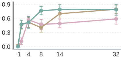
Qwen3
