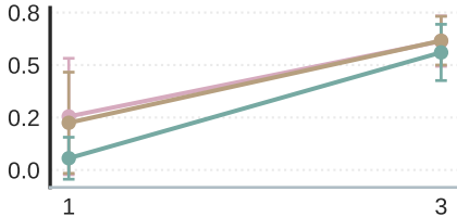
Llama 3.2
