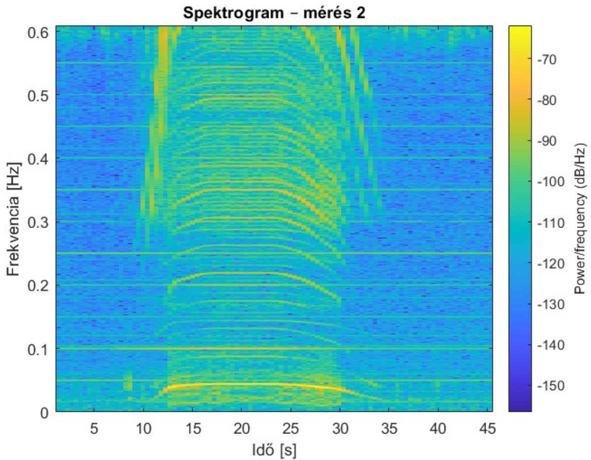
8. ábra. A ventilátor rezgésének spektrogramja
