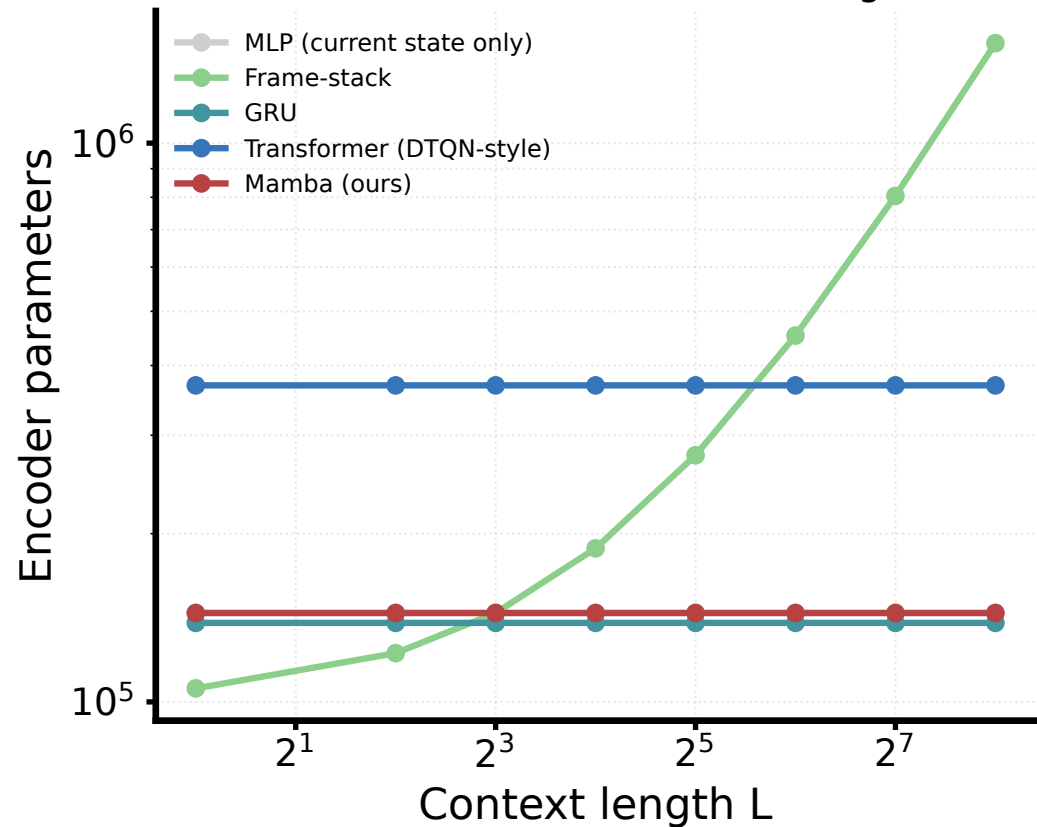
Parameter count vs context length
