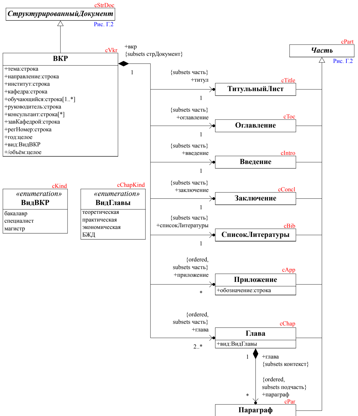
Рис. Г.7 — Выпускная квалификационная работа
