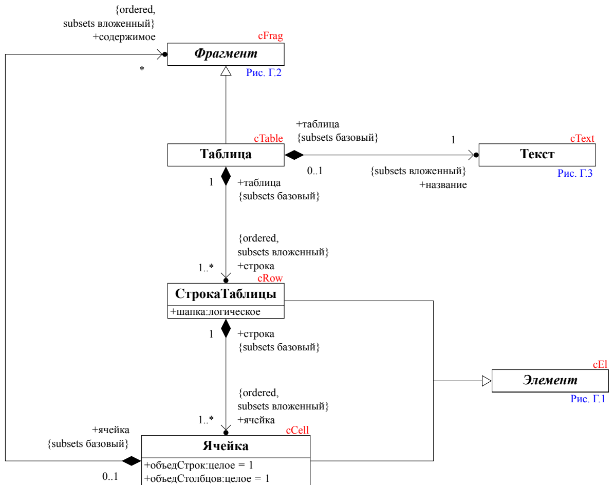
Рис. Г.5 — Фрагмент «таблица»
