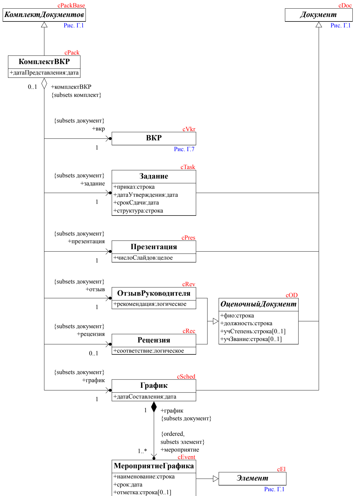
Рис. Г.8 — Комплект документов ВКР
