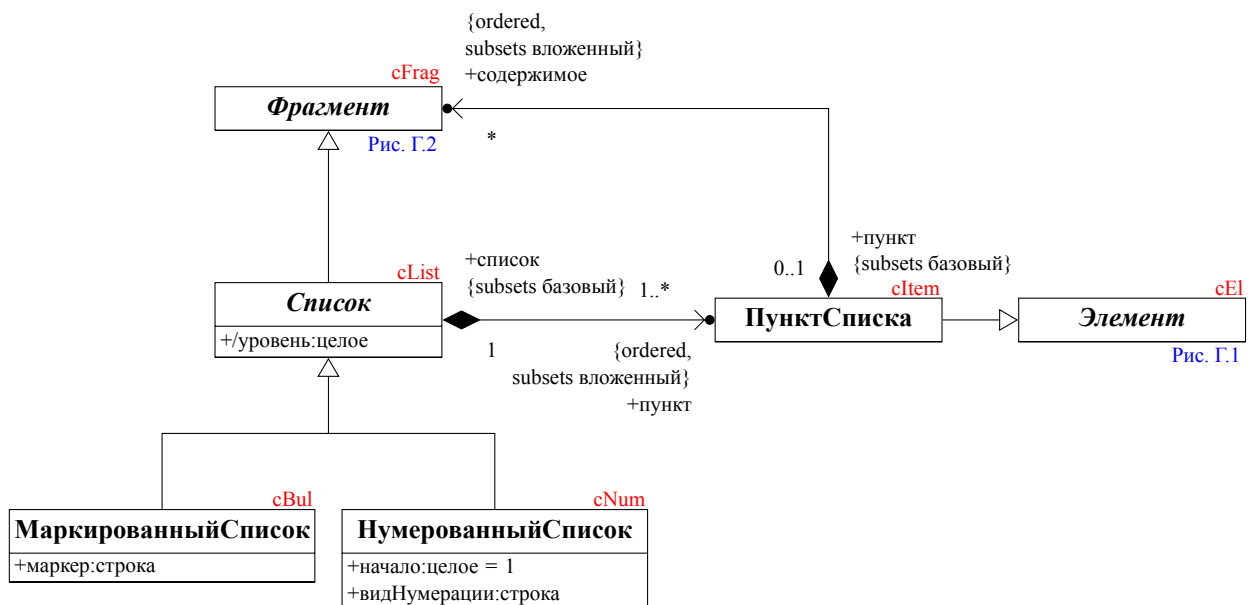
Рис. Г.6 — Фрагмент «список»
