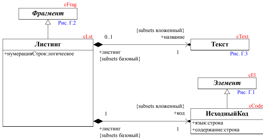
Рис. Г.4 — Фрагмент «листинг»
