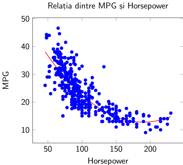
Figure: Task 5: Graficul MPG si Horsepower cu regresie
