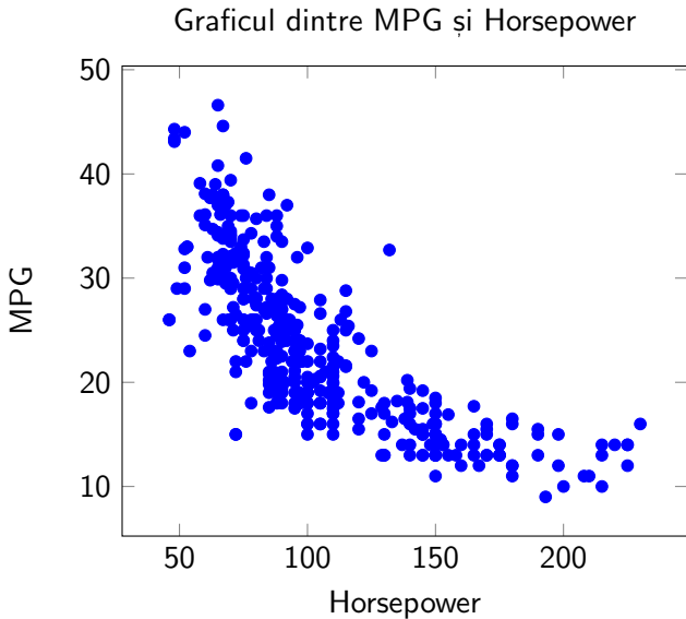
Figure: Task 4: Graficul dintre MPG si Horsepower
