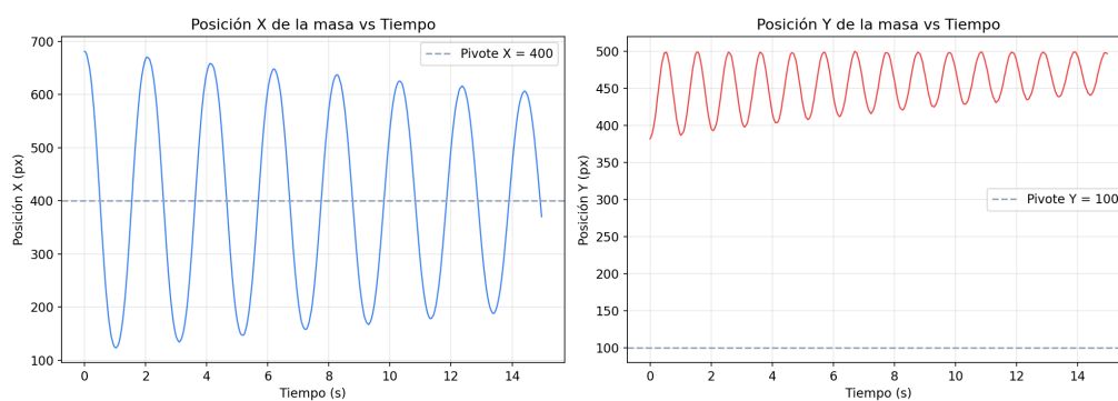
Figura 1: Posición X(t) e Y(t) de la masa del péndulo extraídas del video.
