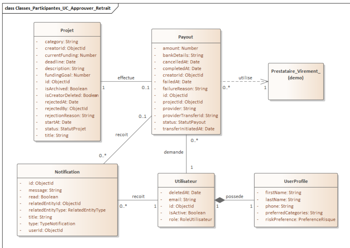
FIGURE 3.12 – Diagramme de classes participantes – Approuver un retrait (Admin)
