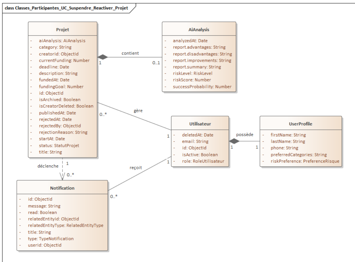
FIGURE 3.14 – Diagramme de classes participantes – Suspendre ou réactiver un projet (Admin)
