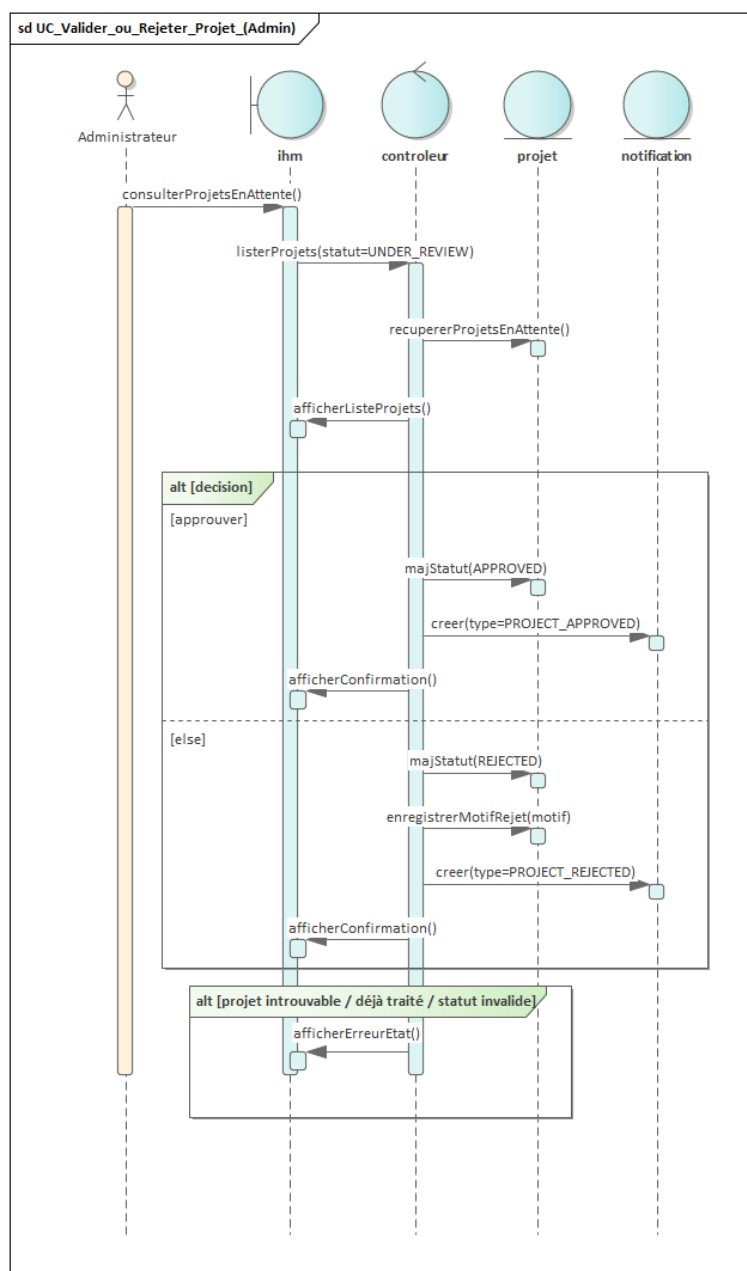
FIGURE 3.7 – Diagramme de séquence – Valider un projet
