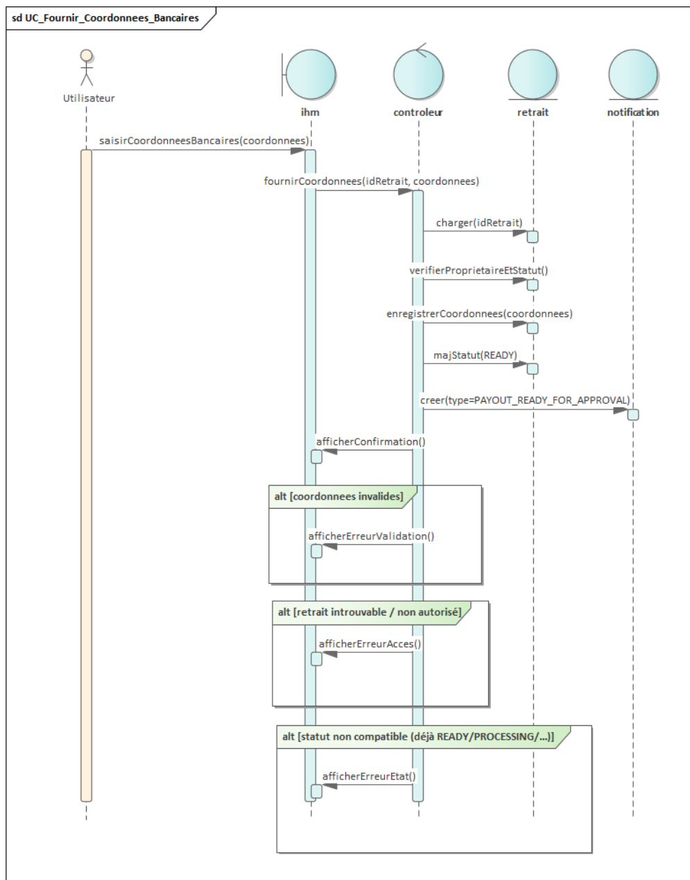
FIGURE 3.9 – Diagramme de séquence – Fournir les coordonnées bancaires
