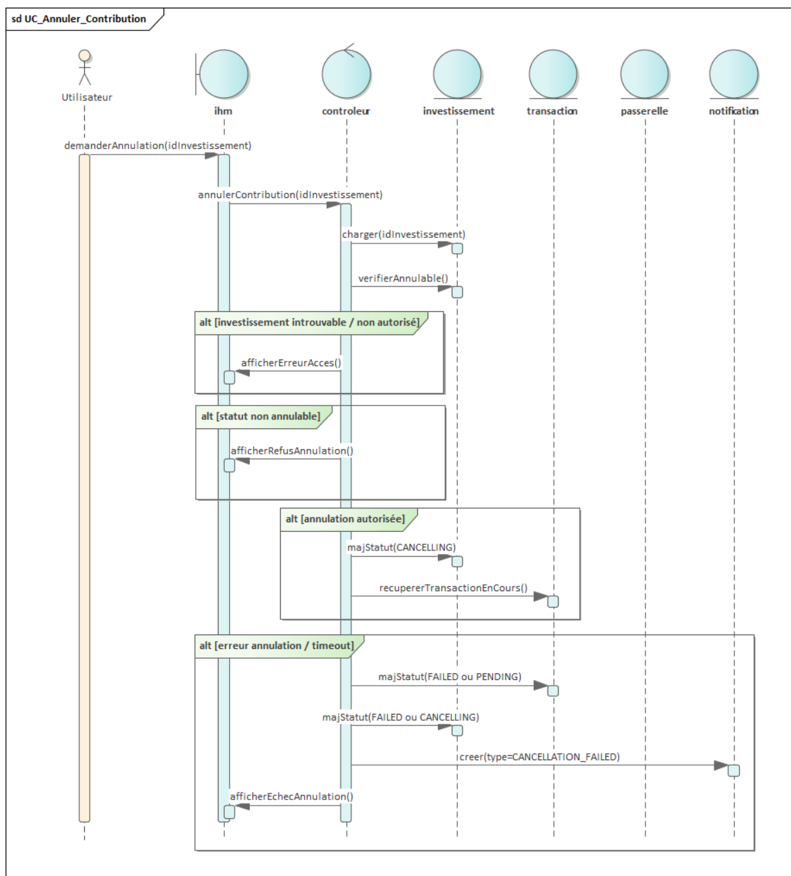
FIGURE 3.1 – Diagramme de séquence – Annuler une contribution
