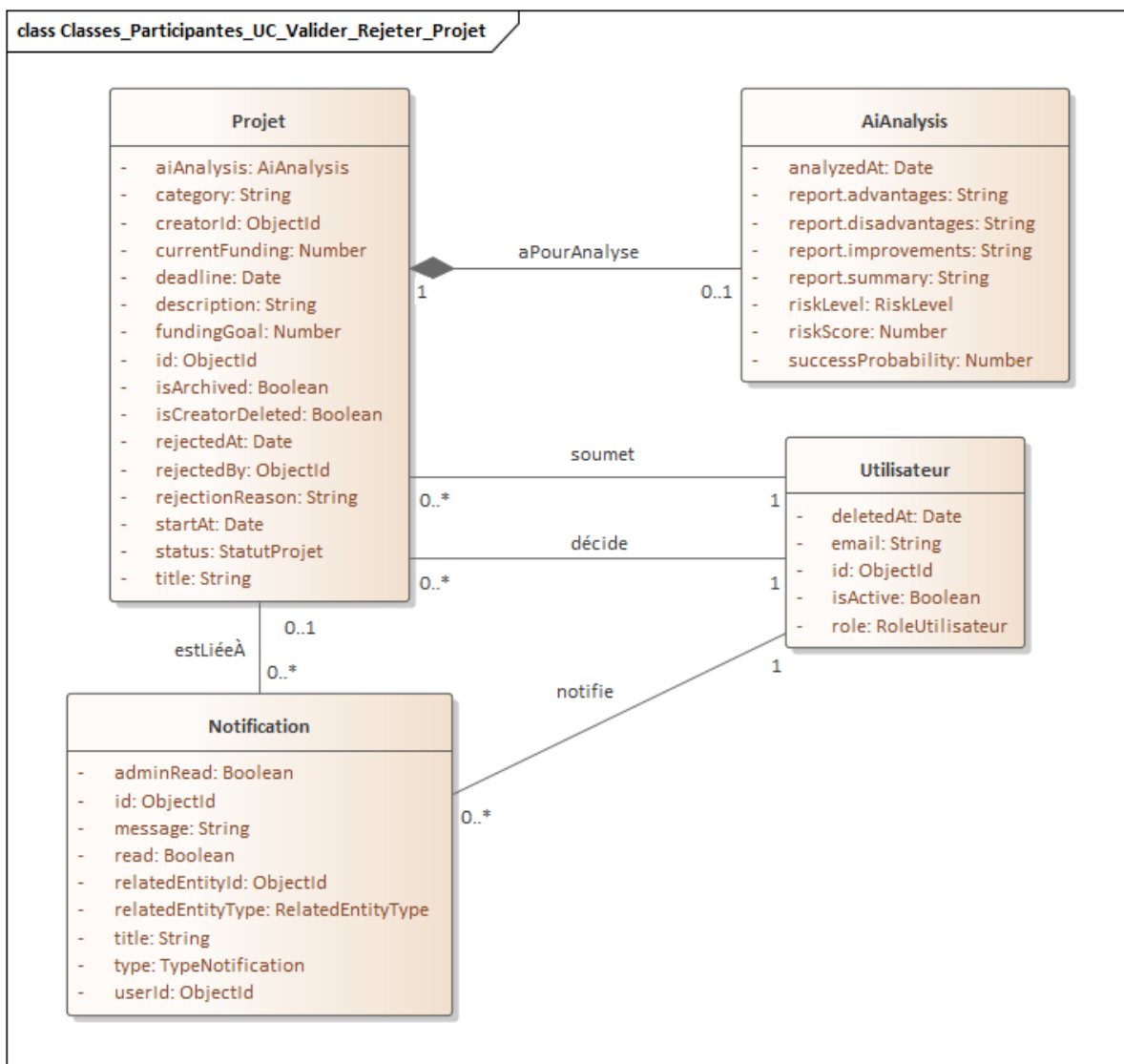
FIGURE 3.8 – Diagramme de classes participantes – Valider ou rejeter un projet (Admin)
