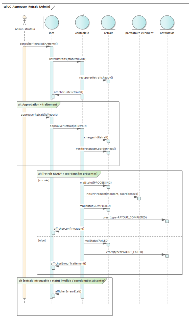
FIGURE 3.11 – Diagramme de séquence – Approuver un retrait (Admin)
