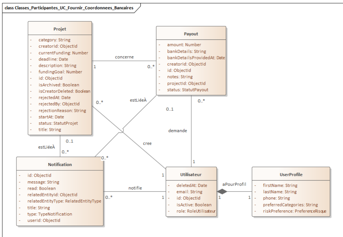
FIGURE 3.10 – Diagramme de classes participantes – Fournir les coordonnées bancaires
