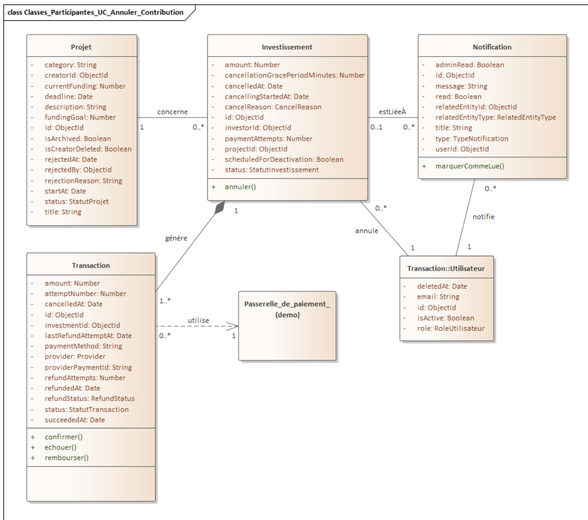
FIGURE 3.2 – Diagramme de classes participantes – Annuler une contribution
