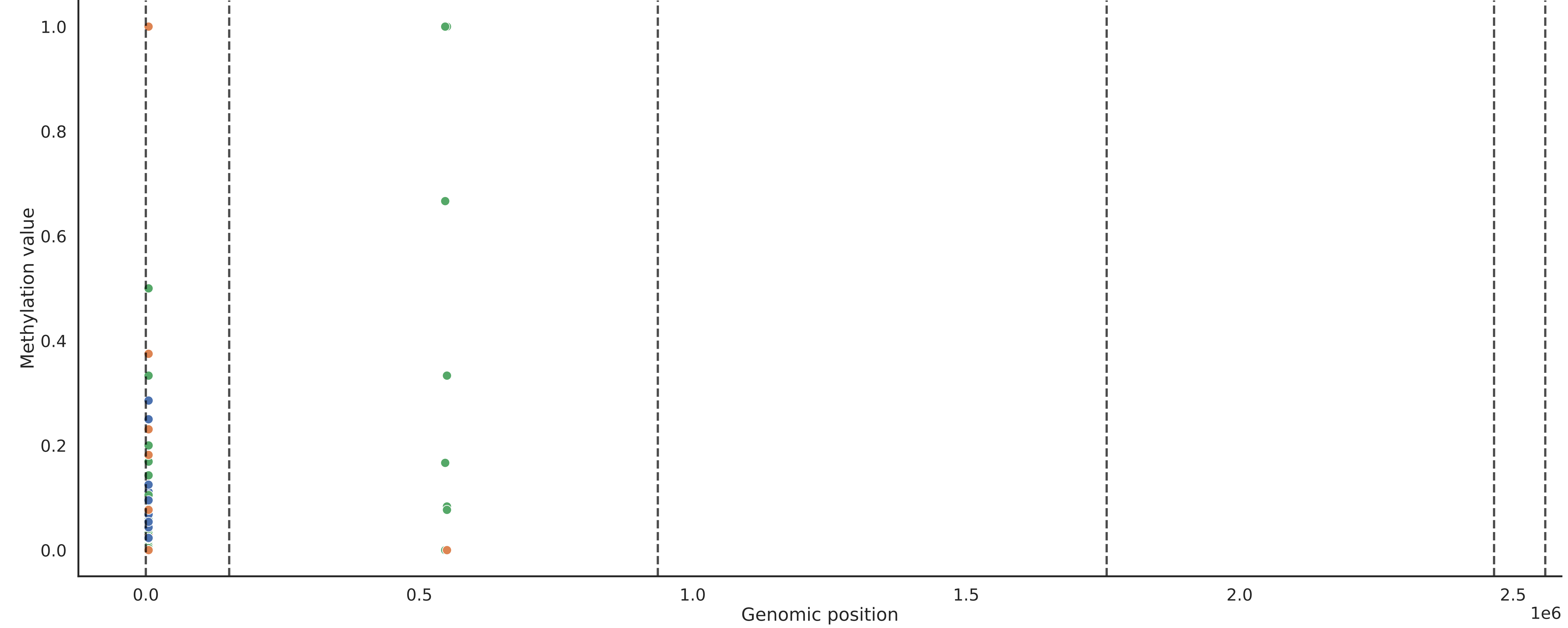
6mA
