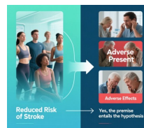
Visual Context
