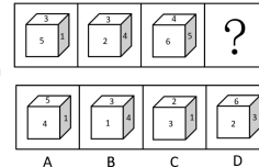
Visual Context
