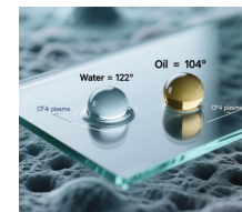
Visual Context
