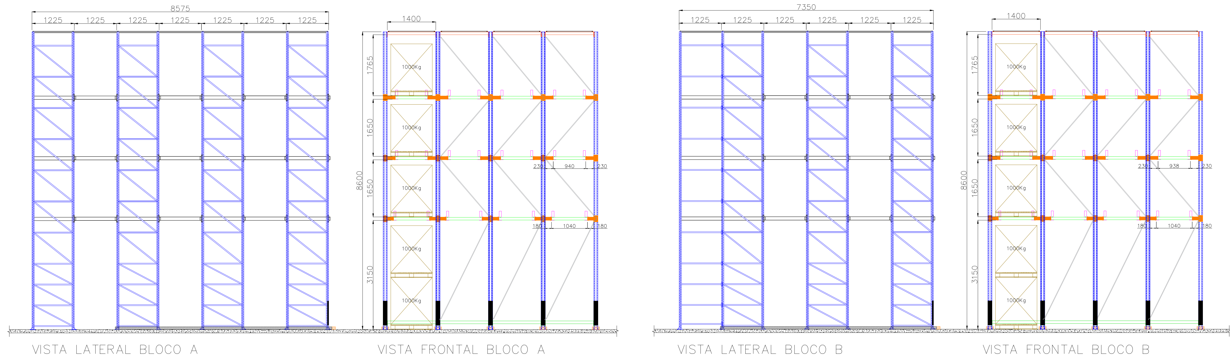
CORTES DRIVE-IN Escala: 1:50
