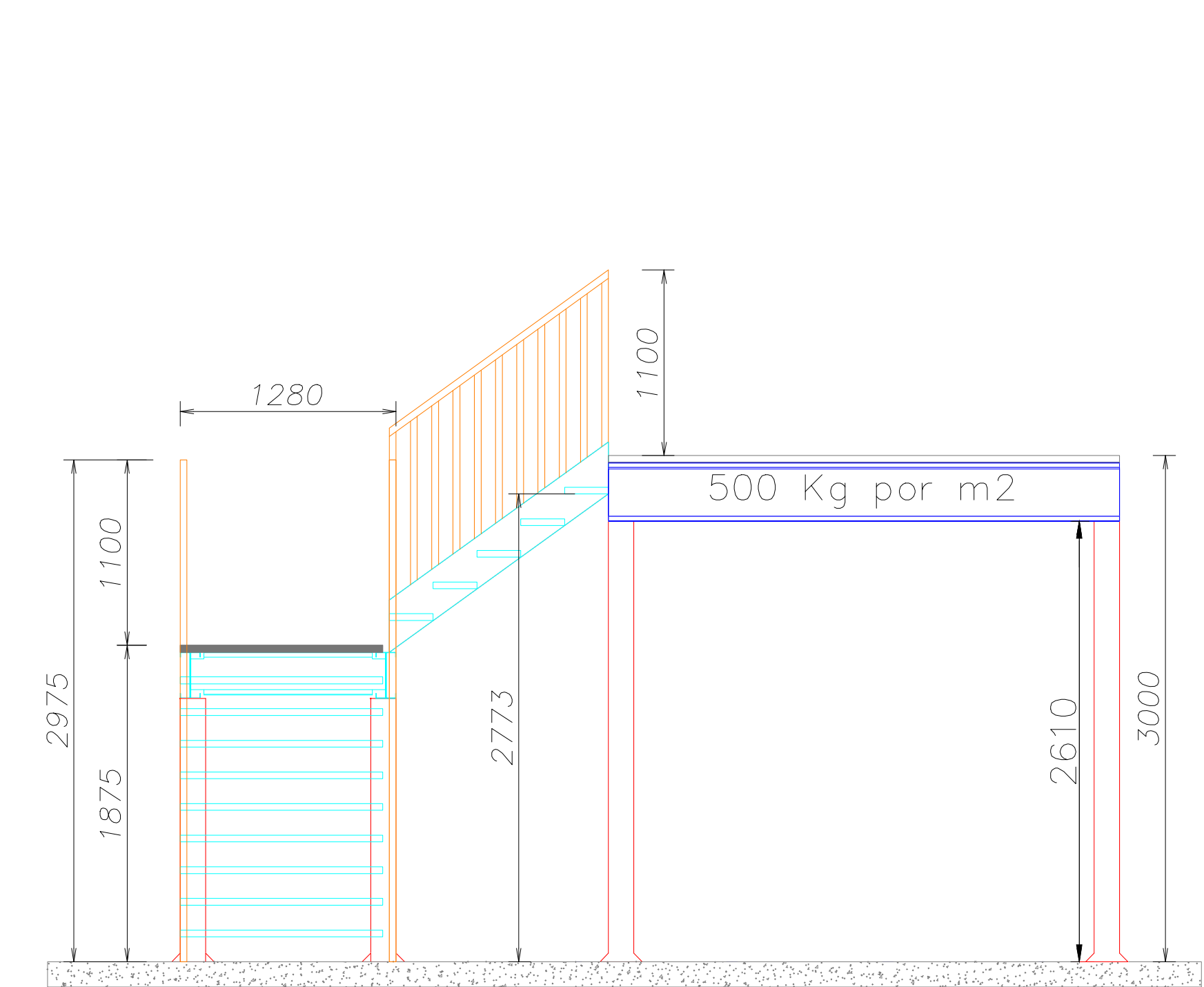
MEZANINO - VISTA LATERAL
