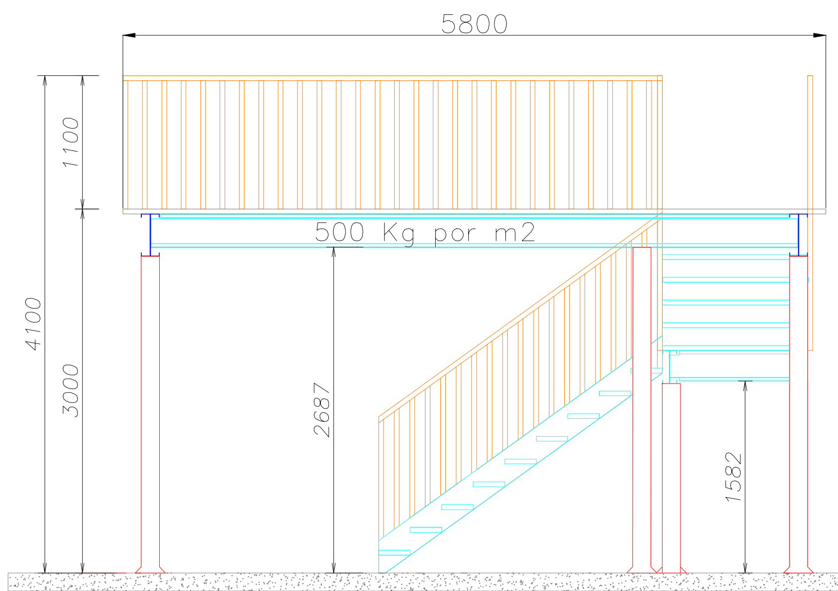
MEZANINO - VISTA FRONTAL
