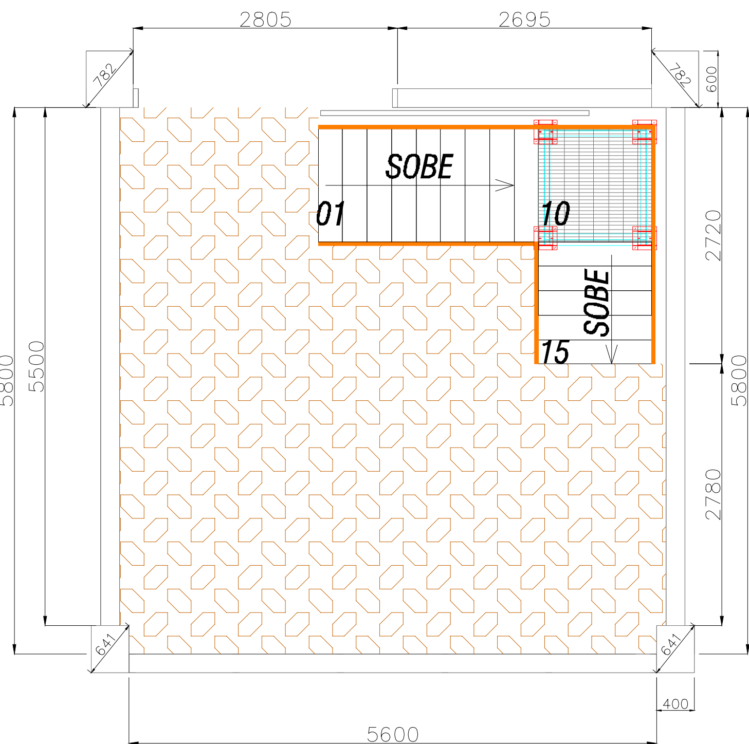
PLANTA BAIXA MEZANINO Escala: 1:125
