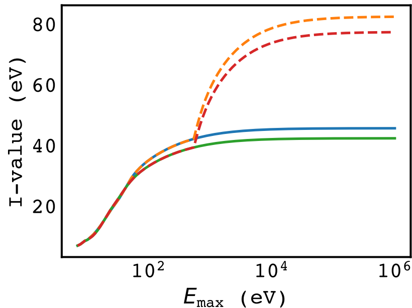
I(E_{\text{max}})
