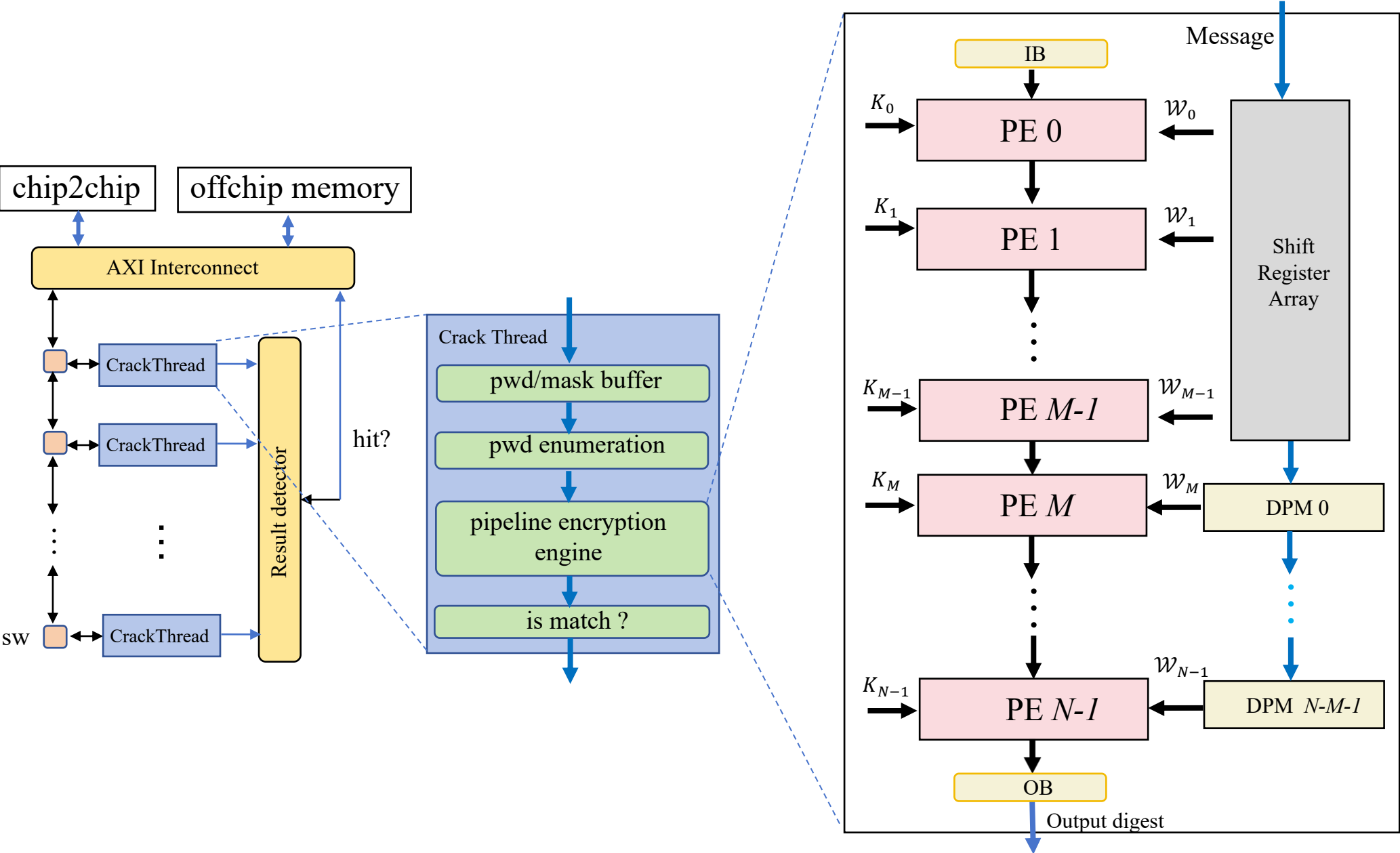
Hash类破译解密构件架构图
