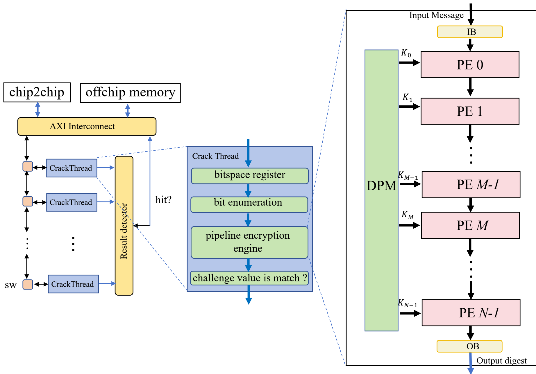
VPN 链路类破译解密构件架构图
