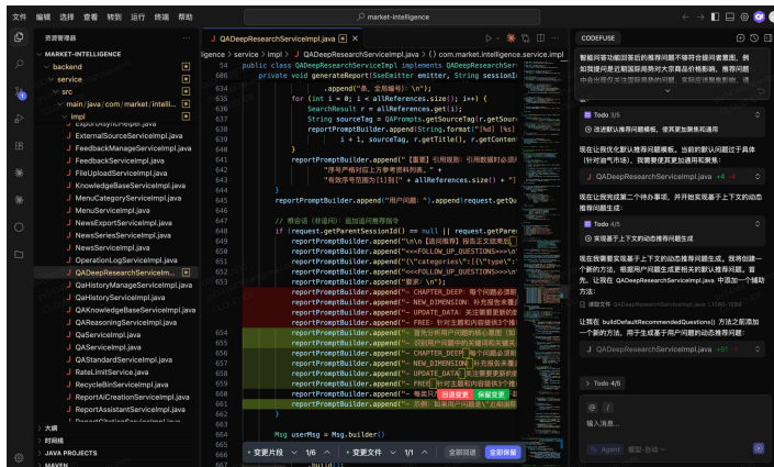
CodeFuse IDE/插件
