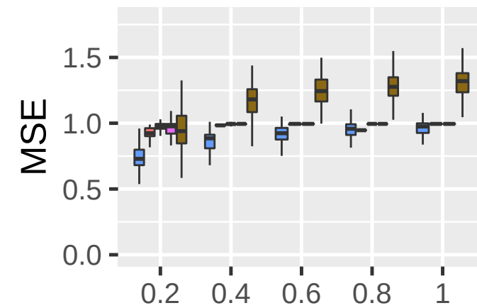
Hyperbola
