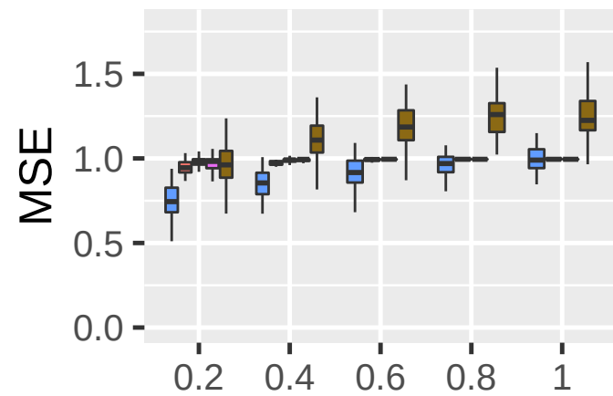
Cosh
