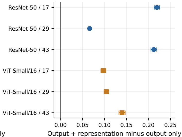
Incremental AUROC
