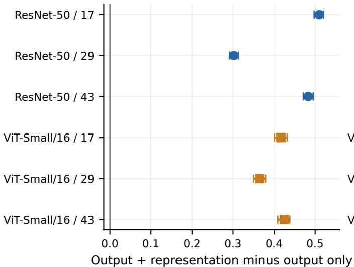
Incremental AP
