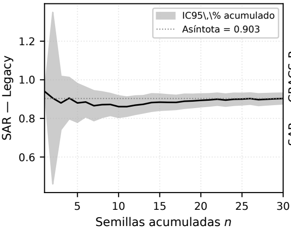
(a) E1, K = 100
