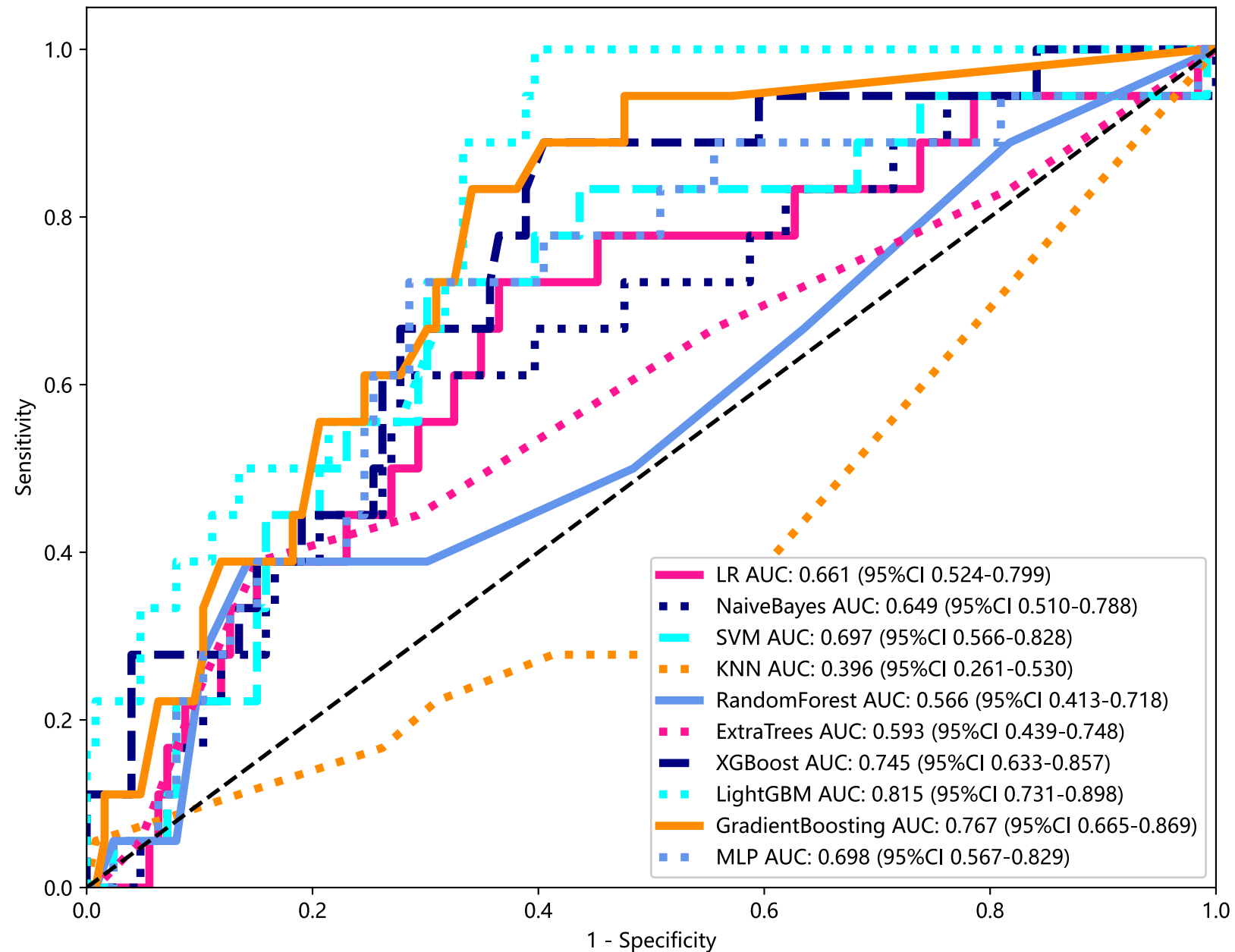
Model AUC
