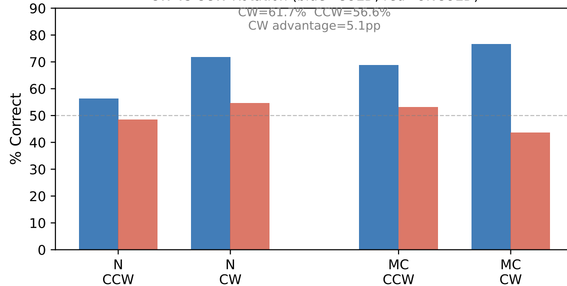
CW vs CCW Rotation (blue=CUED, red=UNCUE)
