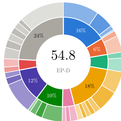
kNN baseline
