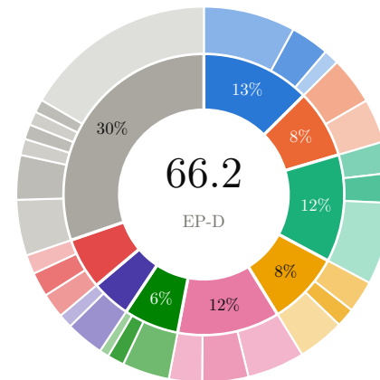
Gemini-3.1-Pro
